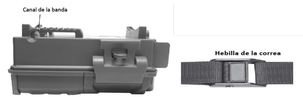
Fig. 5 Fijación de la correa
