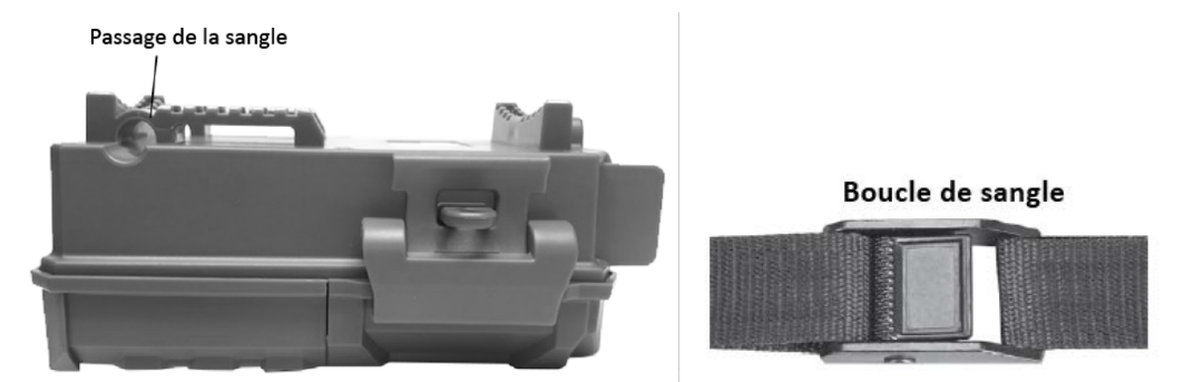
Fig. 5 Fixation de la sangle
