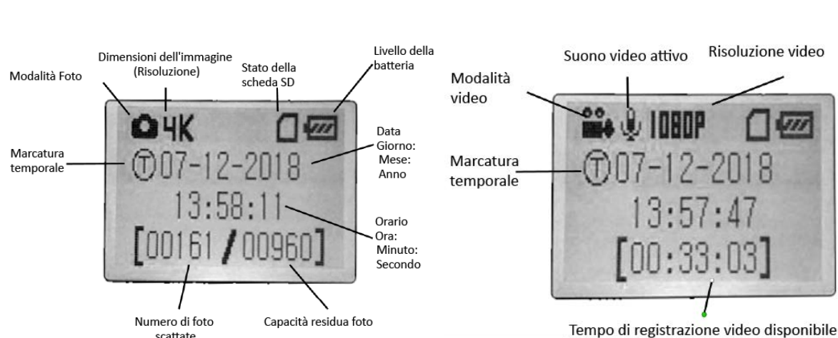
Fig. 3: Schermata informazioni di SETUP (119936C/119938C)
