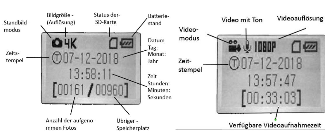
Abb. 3: SETUP-Informationsbildschirm (für die Modelle 119936C / 119938C)
