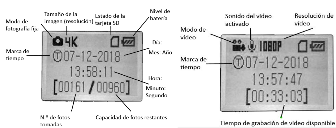
Fig. 3: Pantalla de información de CONFIGURACIÓN (119936C/119938C)
