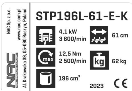
Tabliczka znamionowa
