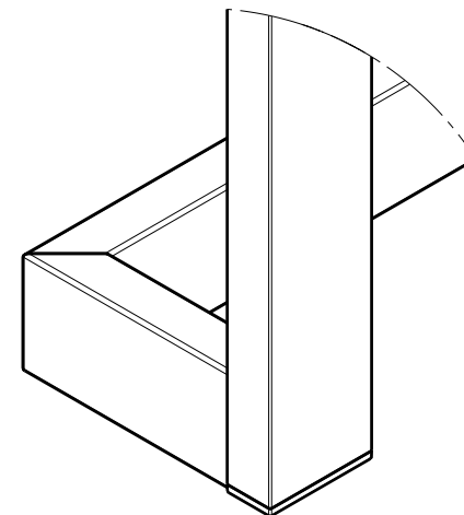
Dettaglio F Scala: 1:2
