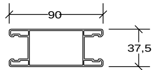
① MONTANT P-MEX 90 X 37,5
