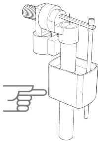
7 Robinet flotteur
