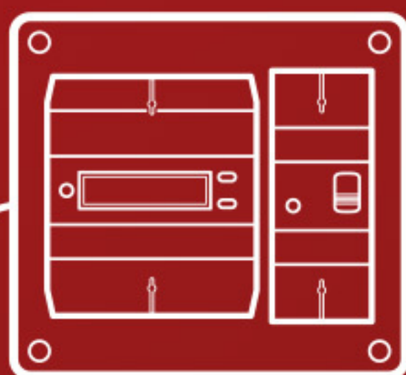
La platine d'abonné EDF (pour disjoncteur général et/ou compteur électronique)
