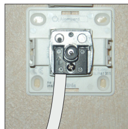
5. Dévisser la bride et mettre en place le câble coaxial
