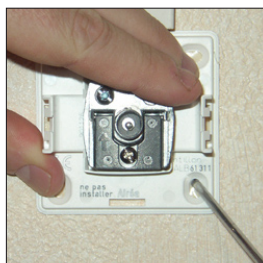
4. Fixer la prise TV
