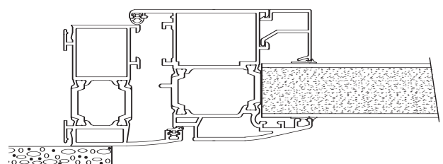
Pose en applique
