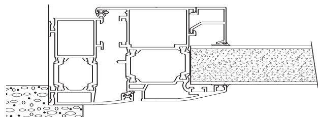
Pose en feuillure
