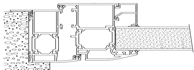
Pose en feuillure afileurant
