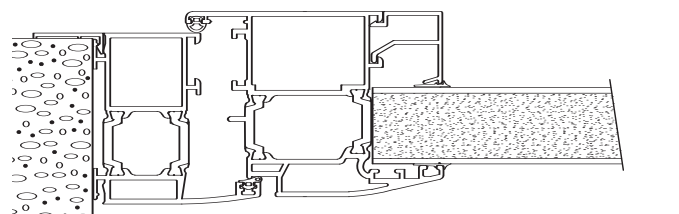
Pose en tunnel afileurant
