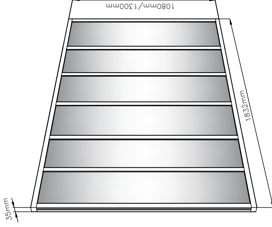
Dimensions de la verrière
