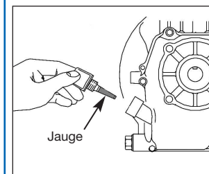
Huile moteur
