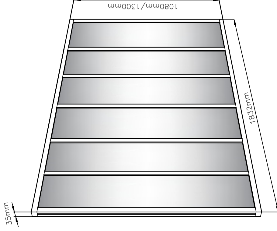
Dimensions de la verrière
