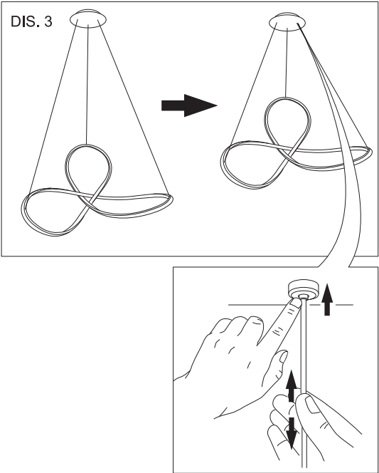
DIS. 3 Regolazione altezza sospensione. Premere il tubetto cromato sporgente per consentire lo scorrimento del cavo, e regolare l'altezza della lampada.
