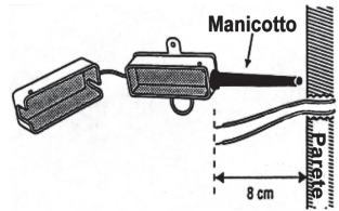
DIS. 1 / DIS. 2 Schema collegamento elettrico alla rete.
