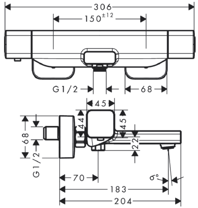
Rysunek wymiarowy
