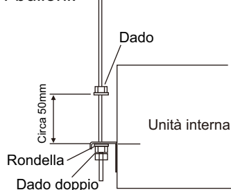
Fig. 3.5 Bulloni e dadi di sospensione
