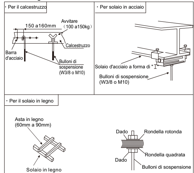
Fig. 3.5 Fissaggio dei bulloni di sospensione
