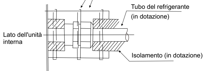
Fig. 4.4 Procedura di isolamento dei tubi
