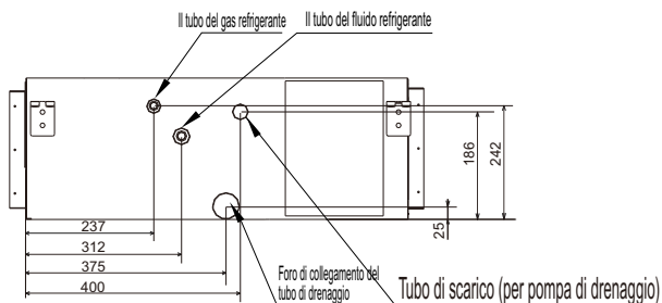
Fig. 4.1 La posizione di connessione del tubo (Unità: mm)
