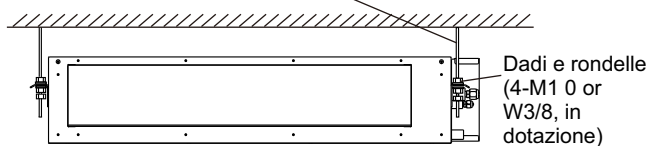
Fig. 3.4 Installazione dell'unità interna
