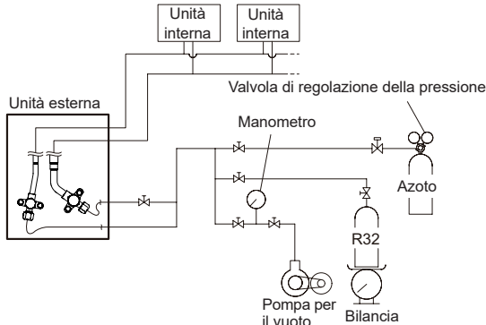
Fig. A Sistema di collegamento
