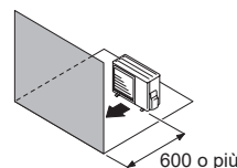
(3) Ostacoli nella parte anteriore
