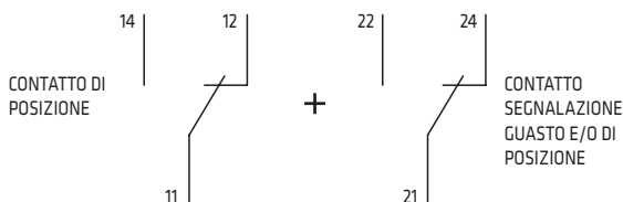
CONTATTO DI SEGNALAZIONE GUASTO E/O POSIZIONE GW 96 765
