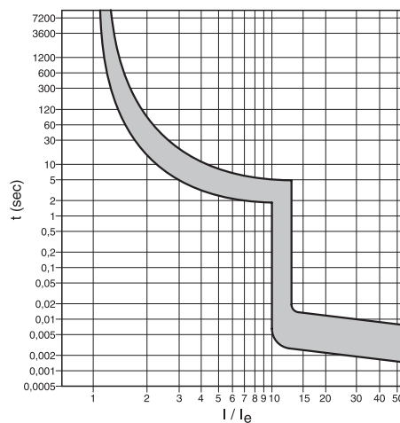
CURVA D'INTERVENTO SALVAMOTORE 1/1,6/2,5/4/6,3/16/25/40A
