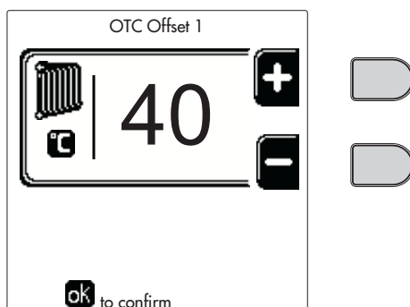
fig. 28- Deplasarea paralelă a curbelor
