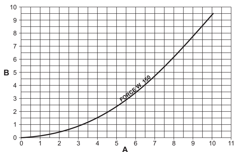
fig. 73- Diagrama de pérdida de carga modelos FORCE W 150
