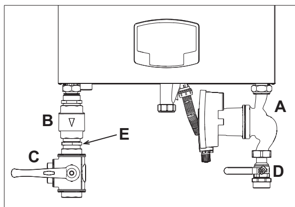
wygląd 36- Kocioł z zainstalowanymi zestawami
