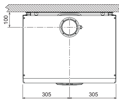
fig. 64 - Vista dall'alto
