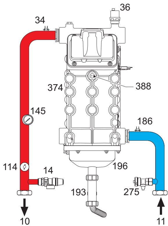
fig. 71- Circuito de agua
