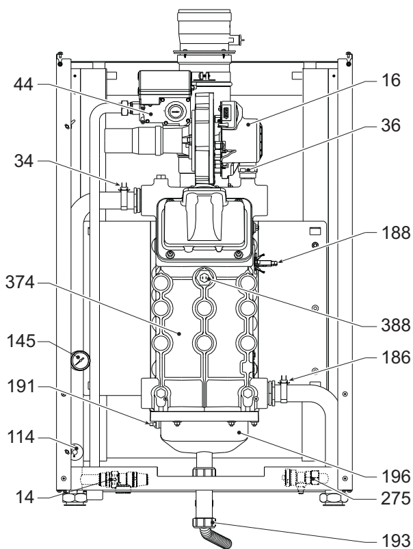
рис. 68- Общий вид, мод. FORCE W 60 и FORCE W 80
