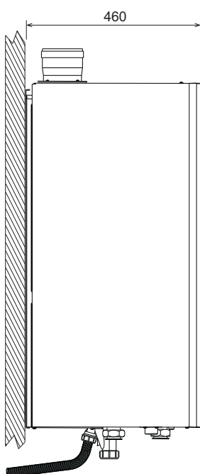
fig. 63- Vedere laterală
