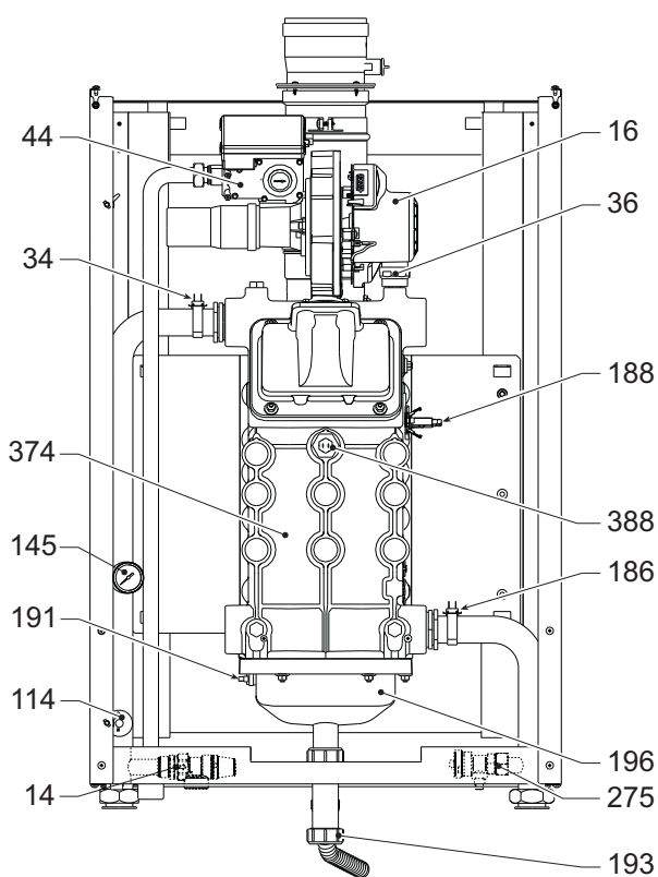
wygląd 68- Widok ogólny mod. FORCE W 60 i FORCE W 80
