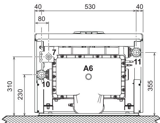
fig. 67- Vedere de jos, mod. FORCE W 150
