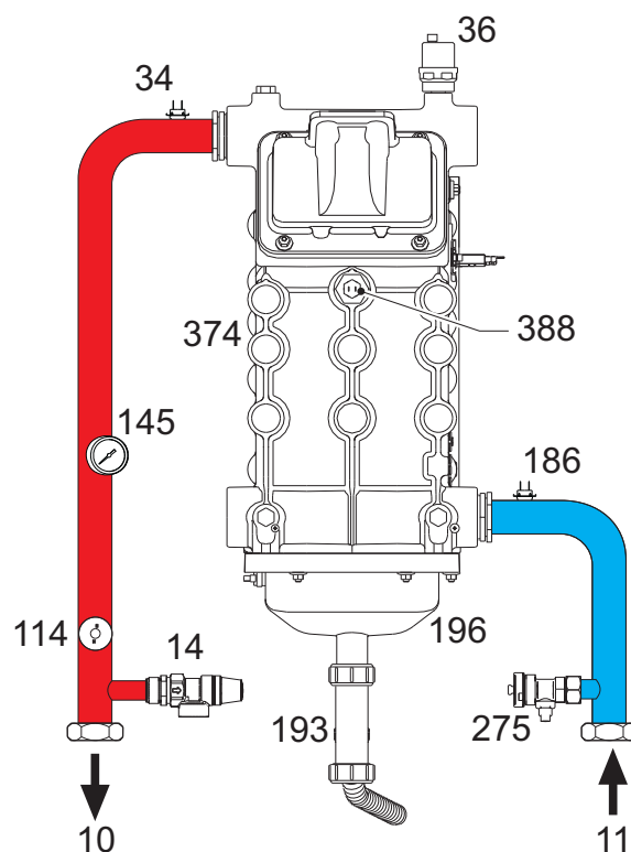
wygląd 71- Obwód hydrauliczny
