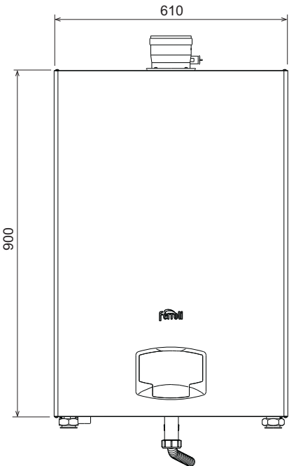
fig. 62- Vista frontal
