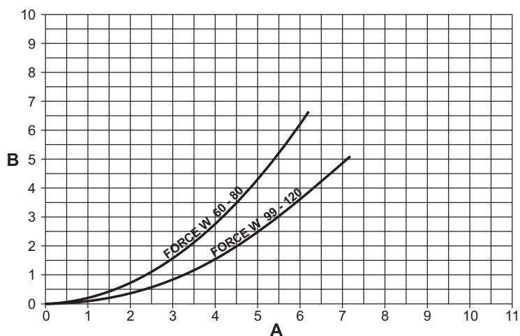
wygląd 72- Wykres strat ciśnienia w modelach FORCE W 60 - FORCE W 80 - FORCE W 99 - FORCE W 120
