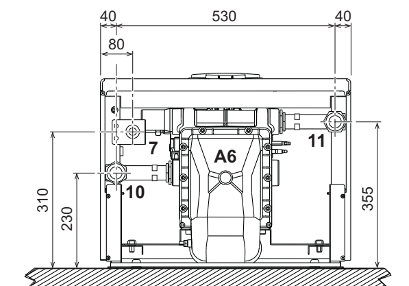
fig. 65 - Vista dal basso mod. FORCE W 60 e FORCE W 80
