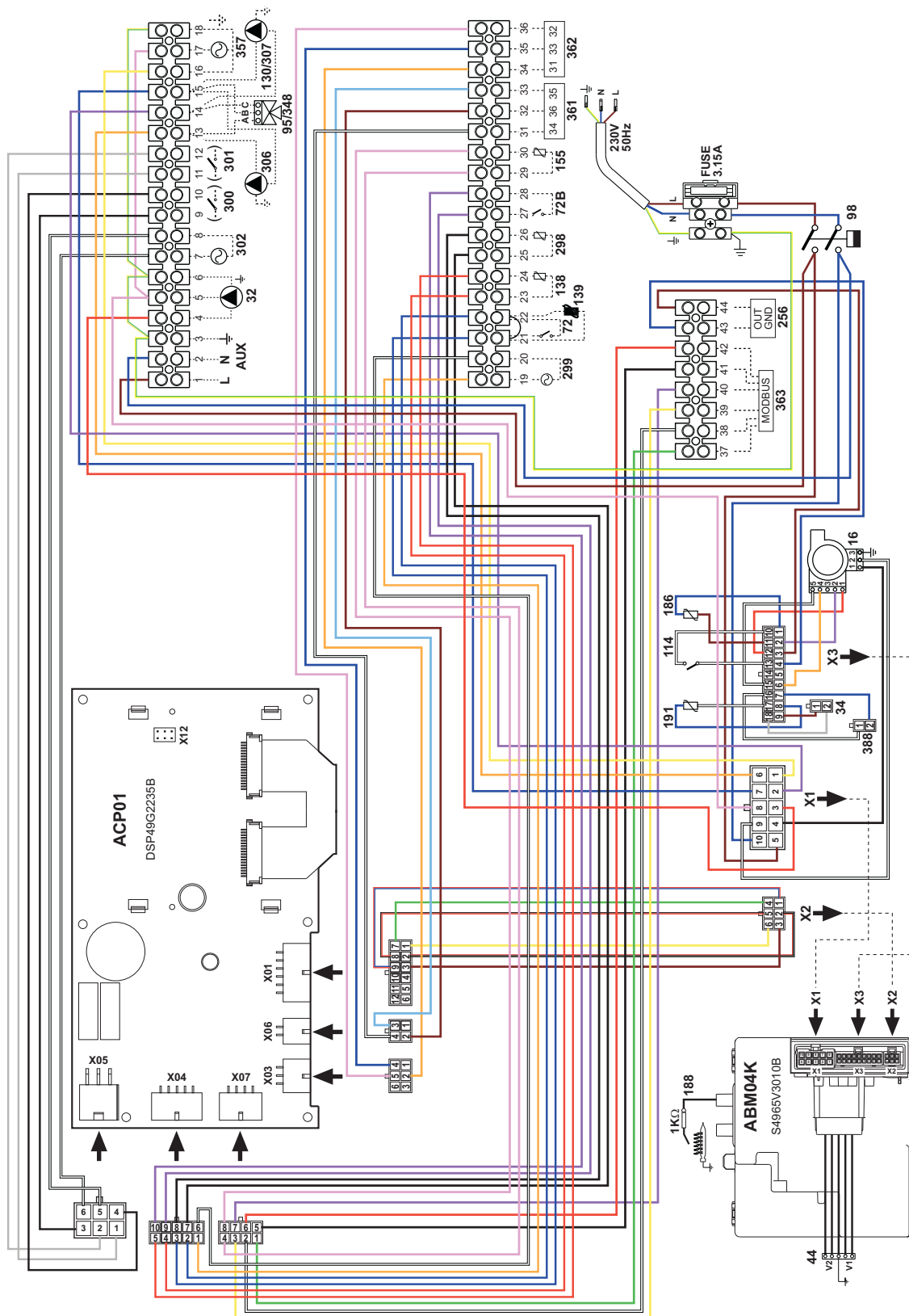
fig. 74 - Schema elettrico modelli FORCE W 60 e FORCE W 80
