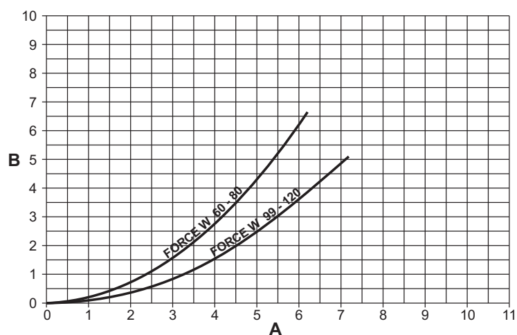
fig. 72- Diagramă pierderi de sarcină modelele FORCE W 60 - FORCE W 80 - FORCE W 99 - FORCE W 120
