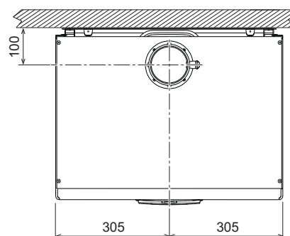
fig. 64- Vedere de sus
