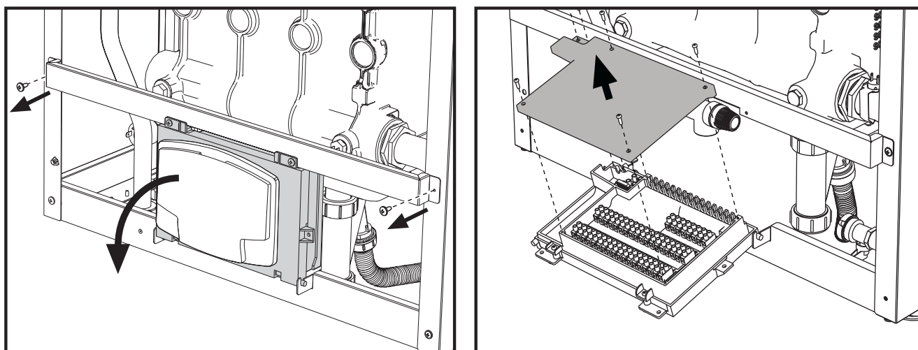
wygląd 53- Elektryczna listwa zaciskowa
