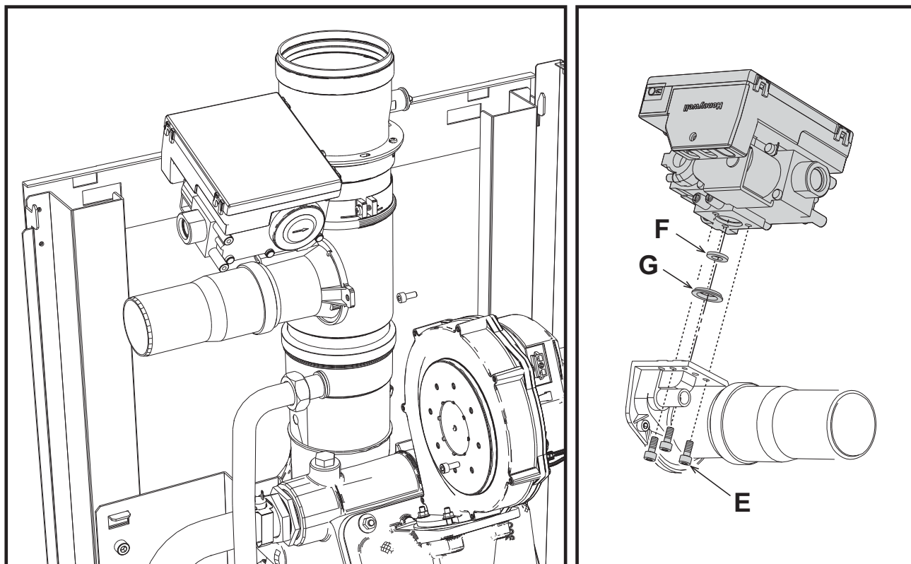
fig. 57 - Modelli FORCE W 60 e FORCE W 80
