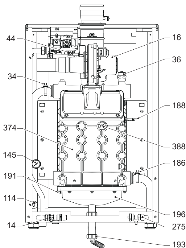
fig. 69 - Vista generale mod. FORCE W 99 e FORCE W 120
