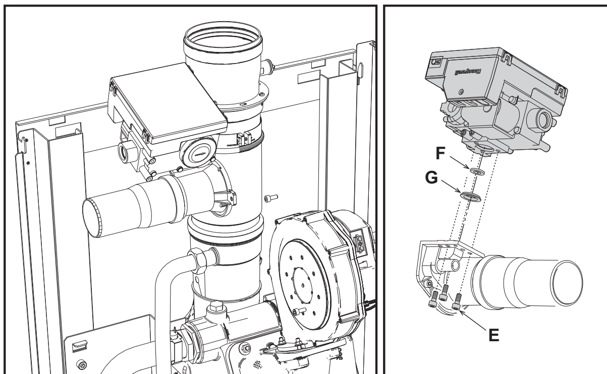
рис. 57- Модели FORCE W 60 и FORCE W 80
