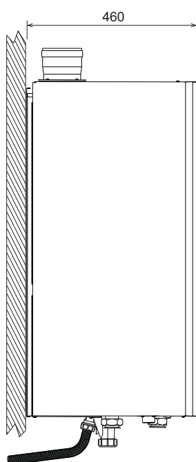
рис. 63- Вид сбоку
