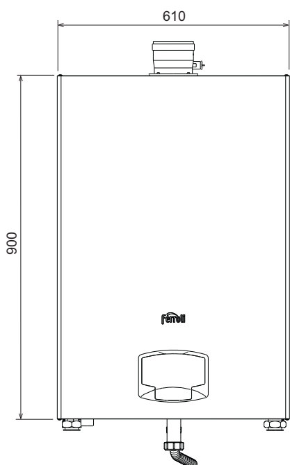
рис. 62- Вид спереди
