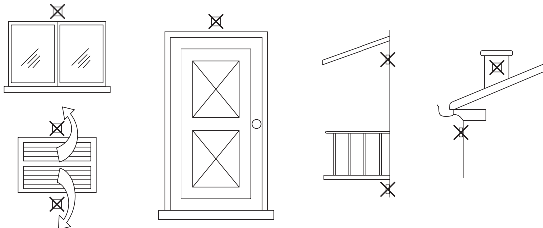
fig. 52 - Poziționare nerecomandată pentru sonda externă
