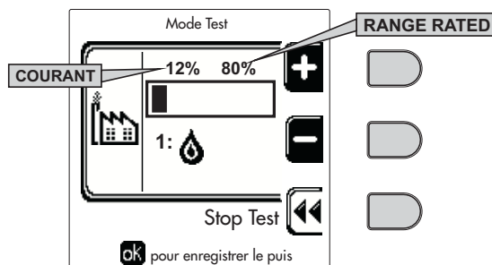
fig. 59 - Mode TEST (exemple puissance chauffage = 80%)
