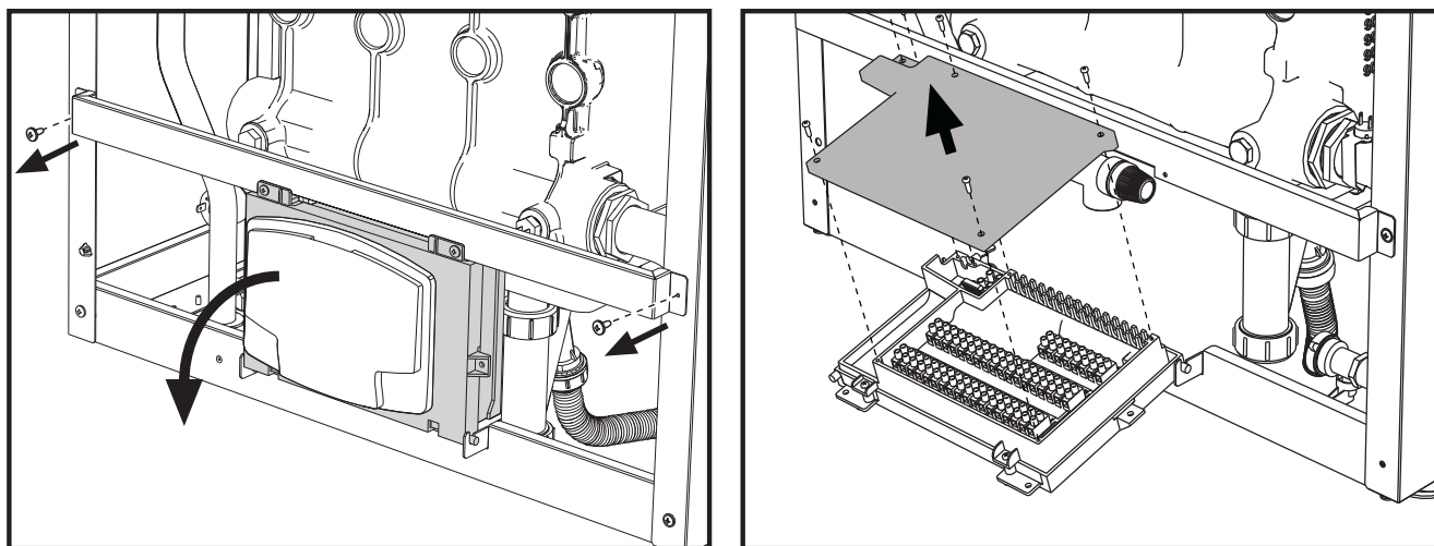
fig. 53 - Morsettiera elettrica
