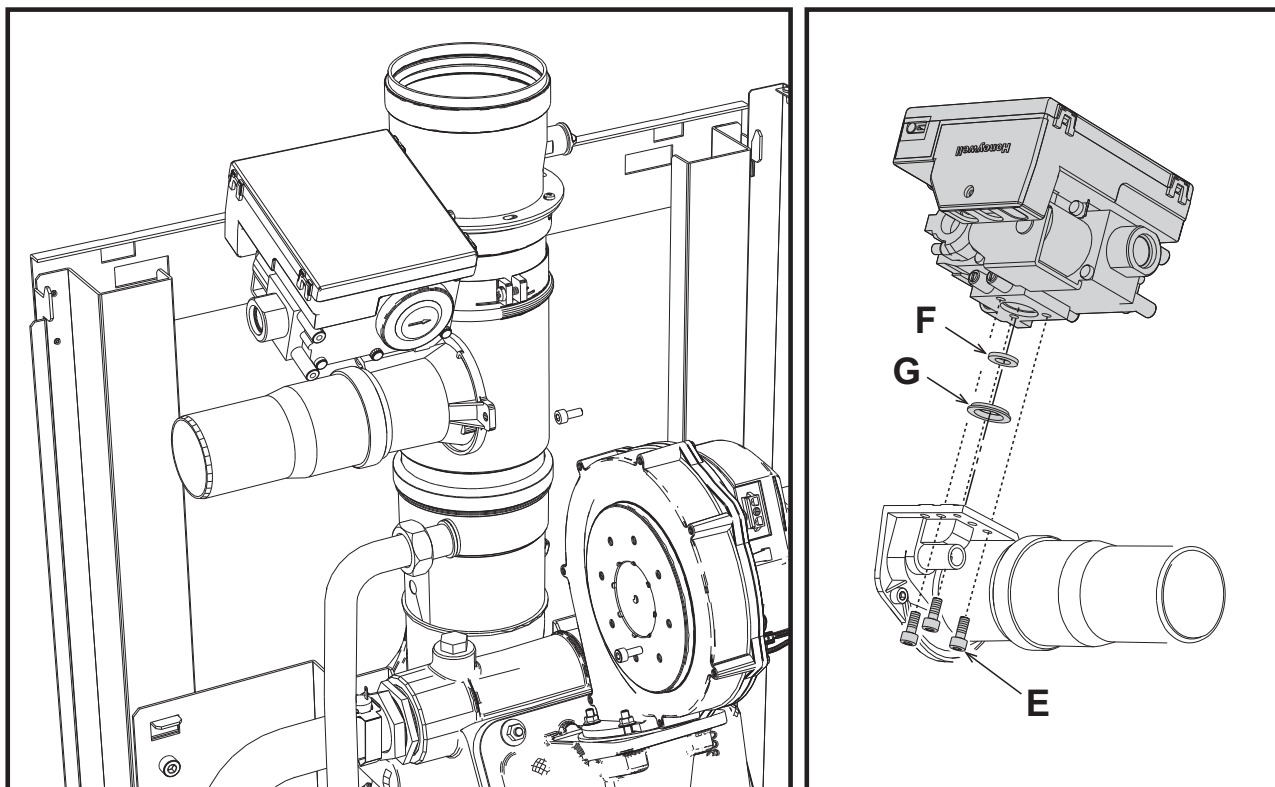
fig. 57- Modèles FORCE W 60 et FORCE W 80
