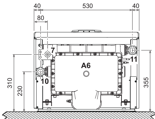
fig. 67- Vue de dessous mod. FORCE W 150
