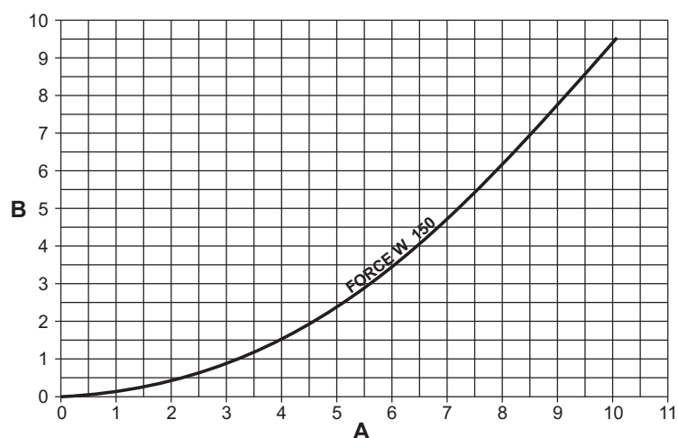
fig. 73- Diagramme perte de charge modèles FORCE W 150
