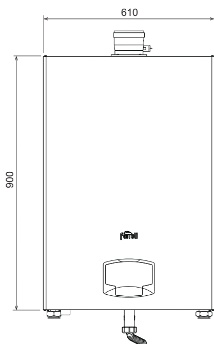
wygląd 62- Widok z przodu
