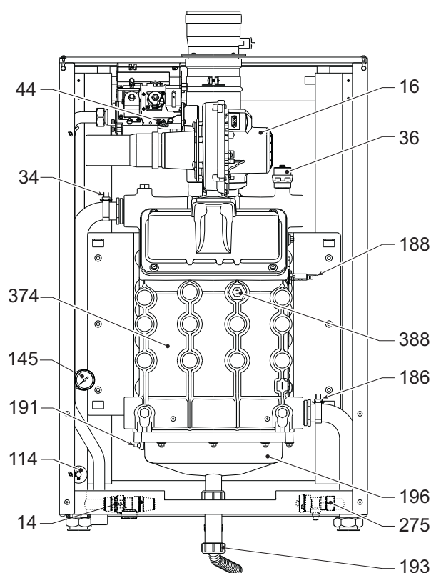
fig. 69- Vue générale mod. FORCE W 99 et FORCE W 120
