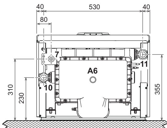
fig. 67 - Vista dal basso mod. FORCE W 150
