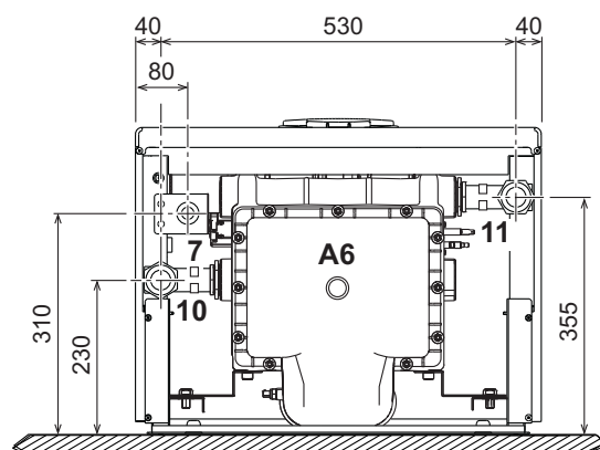
fig. 66- Vedere de jos, mod. FORCE W 99 și FORCE W 120
