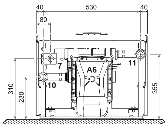
fig. 65- Vedere de jos, mod. FORCE W 60 și FORCE W 80
