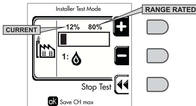
wygląd 59- Tryb TEST (przykład mocy ogrzewania = 80%)
