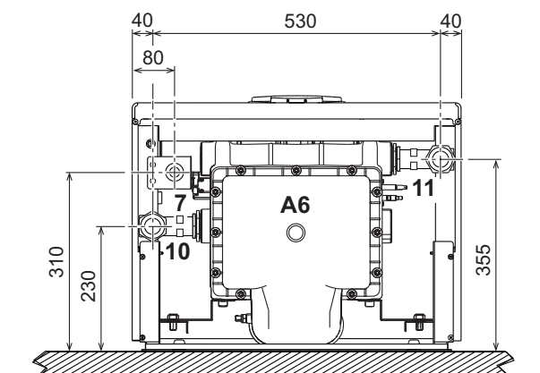
fig. 66 - Vista dal basso mod. FORCE W 99 e FORCE W 120
