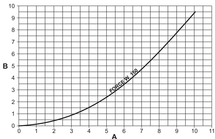
fig. 73 - Diagramma perdita di carico modelli FORCE W 150
