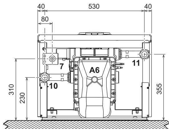
fig. 65- Vue de dessous mod. FORCE W 60 et FORCE W 80
