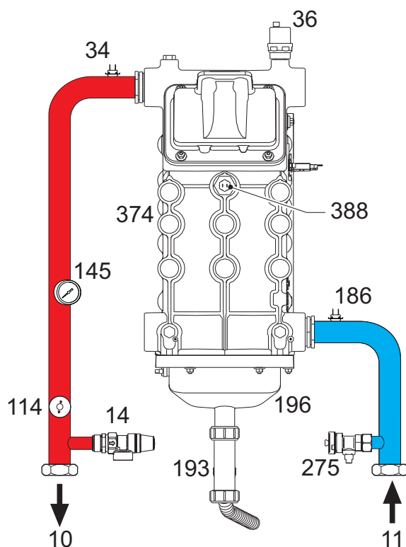
fig. 71- Circuit hydraulique
