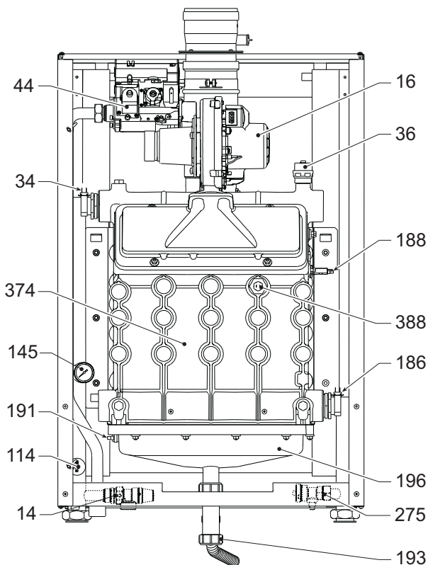
рис. 70- Общий вид, мод. FORCE W 150
