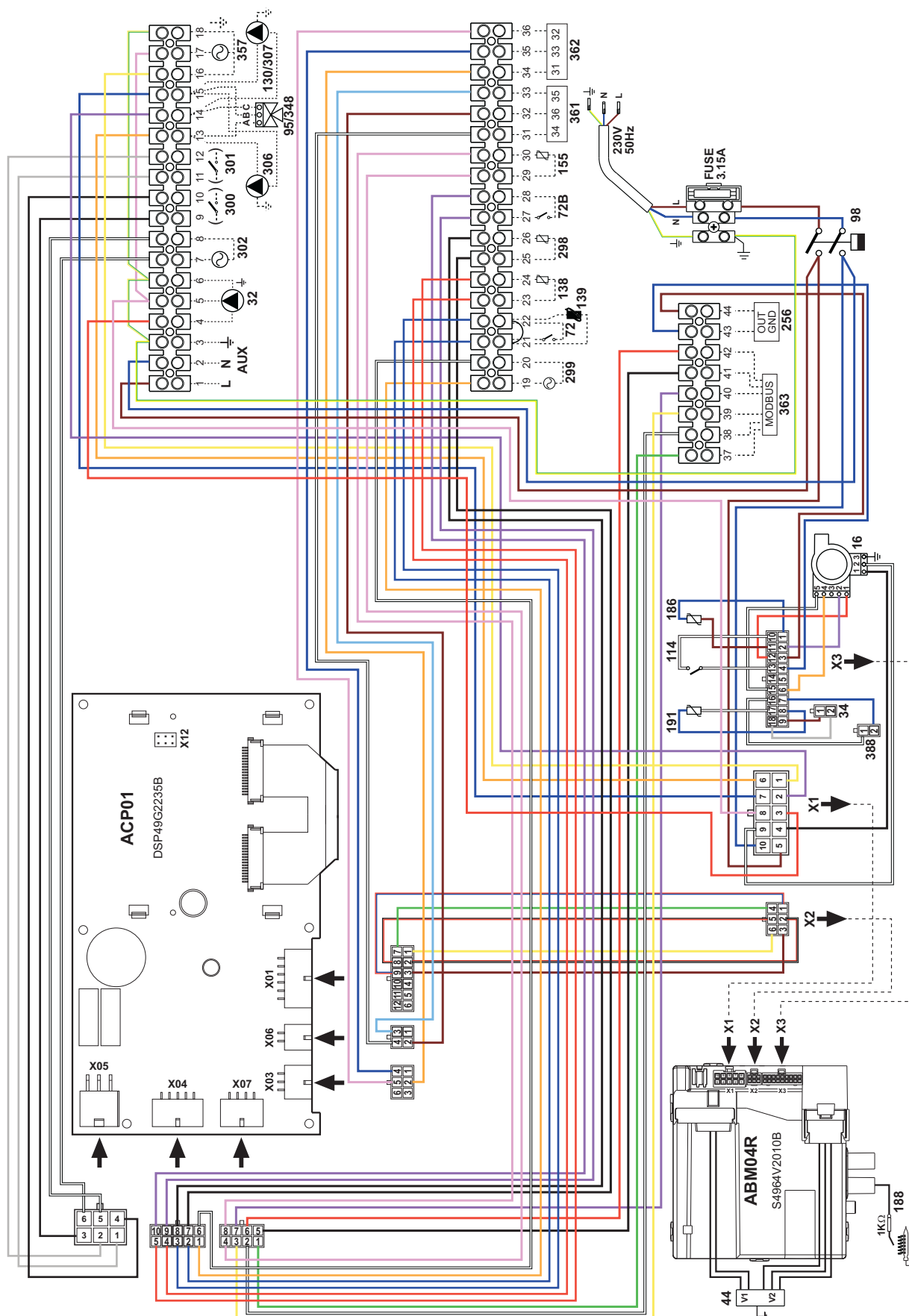
fig. 75- Schemă electrică modelele FORCE W 99, FORCE W 120 și FORCE W 150
