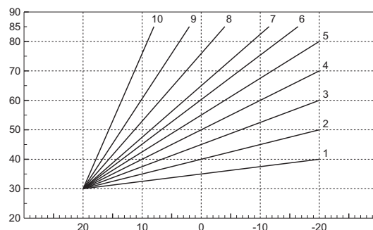
fig. 29 - Curbe de compensare
