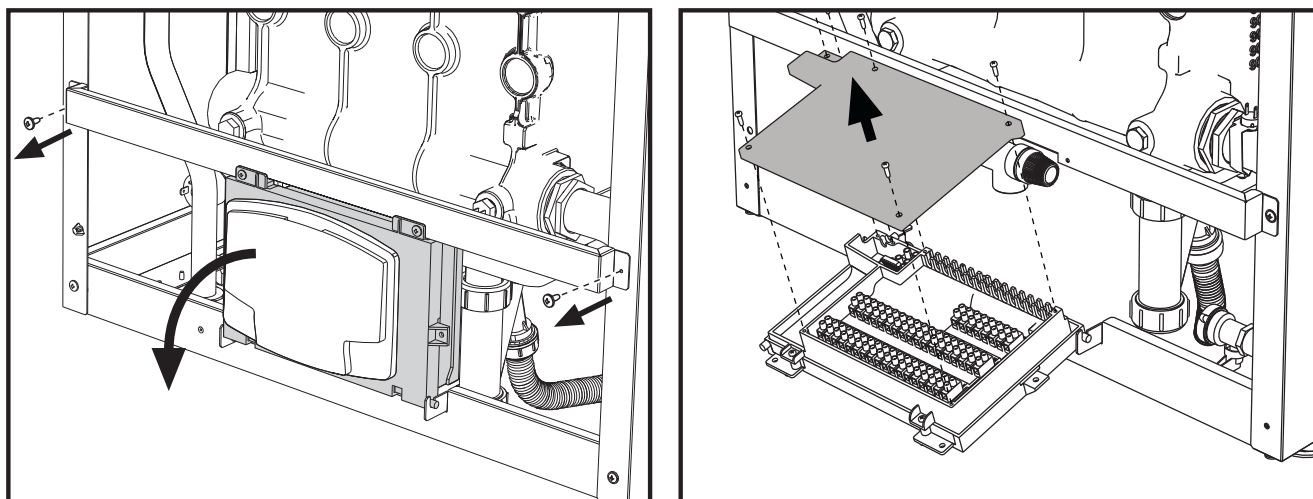
fig. 53- Panoul de borne electric
