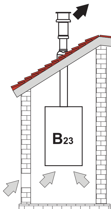
fig. 54- Exemple de conectare (⇨ = Aer / ⇨ = Gaze arse)
