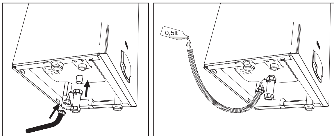
wygląd 55- Podłączenie spustu kondensatu
