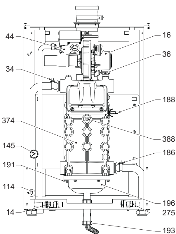
fig. 68 - Vista generale mod. FORCE W 60 e FORCE W 80
