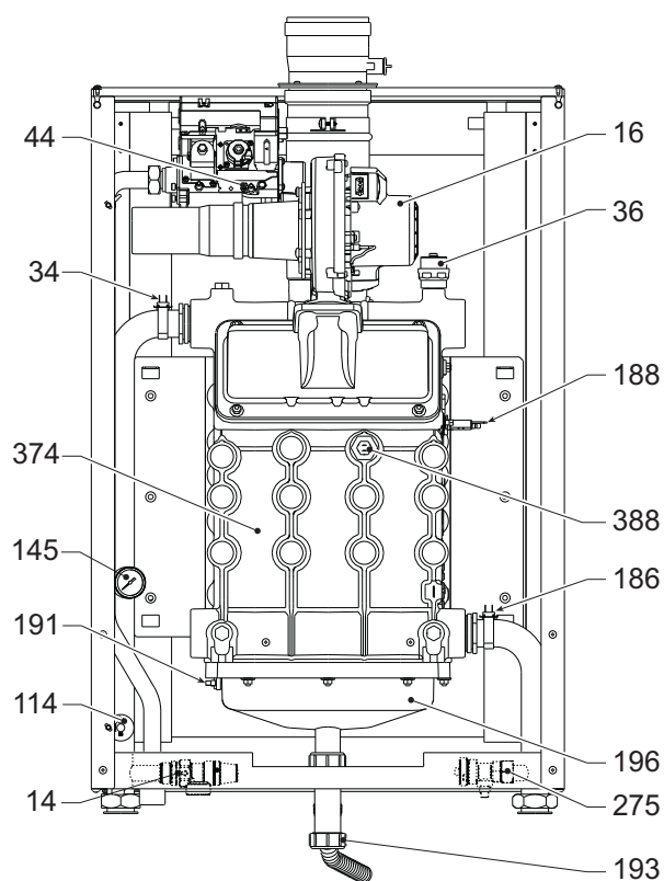
fig. 69- Vedere generală mod. FORCE W 99 și FORCE W 120
