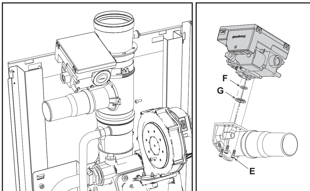
wygląd 57- Modele FORCE W 60 i FORCE W 80
