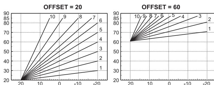
fig. 30- Exemplu de deplasare paralelă a curbelor de compensare
