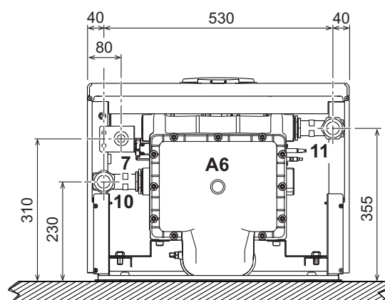
рис. 66- Вид снизу, мод. FORCE W 99 и FORCE W 120
