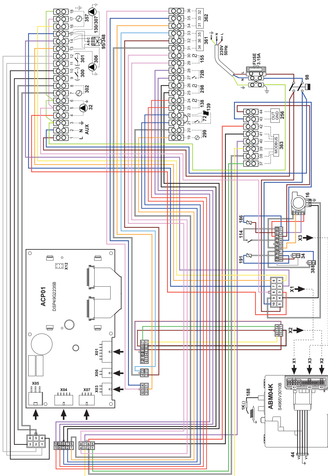
рис. 74- Электрическая схема моделей FORCE W 60 и FORCE W 80
