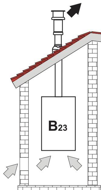
wygląd 54- Przykłady połączenia (⇨ = Powietrze / ⇨ = Spaliny)
