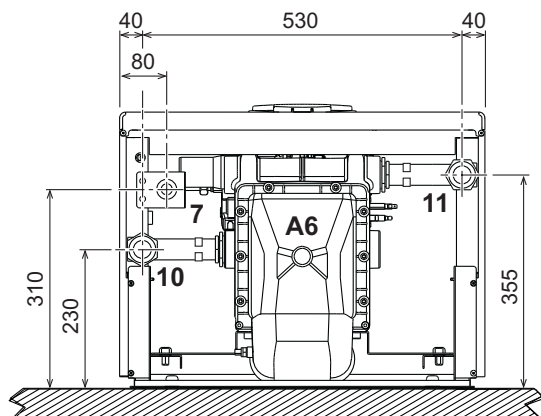
wygląd 65- Widok od dołu mod. FORCE W 60 i FORCE W 80
