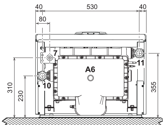
рис. 67- Вид снизу, мод. FORCE W 150
