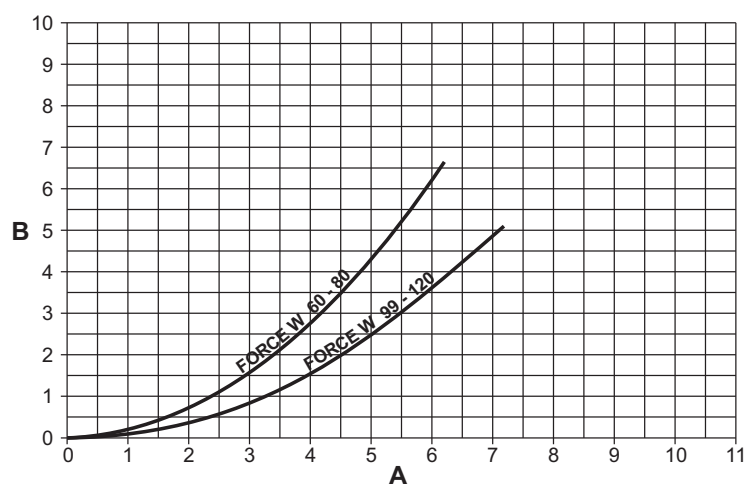
fig. 72- Diagrama de pérdida de carga modelos FORCE W 60 - FORCE W 80 - FORCE W 99 - FORCE W 120
