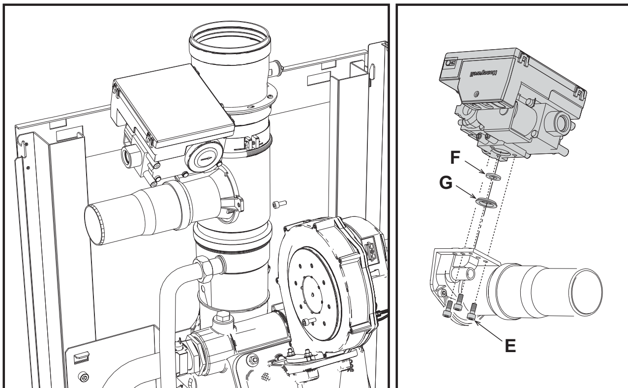
fig. 57- Modelos FORCE W 60 y FORCE W 80
