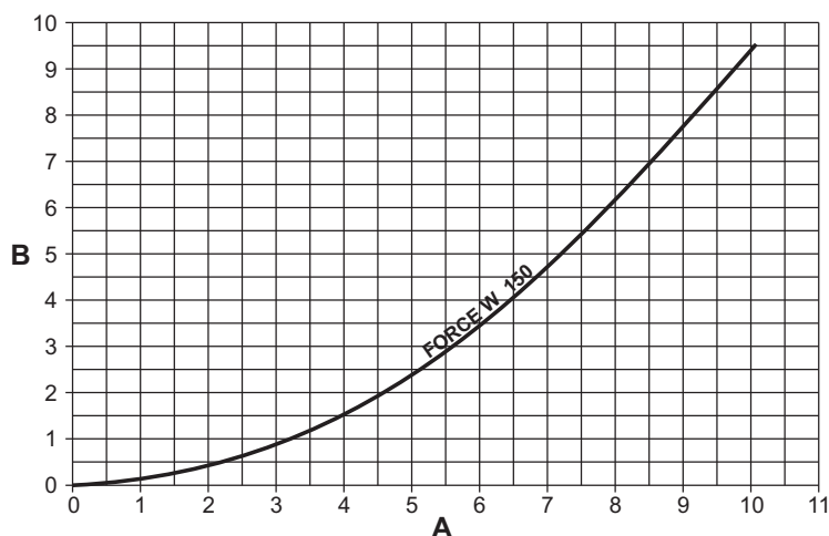
wygląd 73- Wykres strat ciśnienia w modelach FORCE W 150
