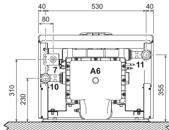
fig. 66- Vue de dessous mod. FORCE W 99 et FORCE W 120
