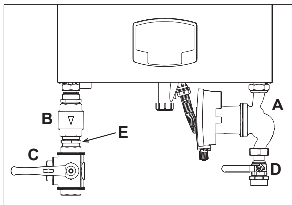
fig. 36- Centrală cu kiturile instalate
