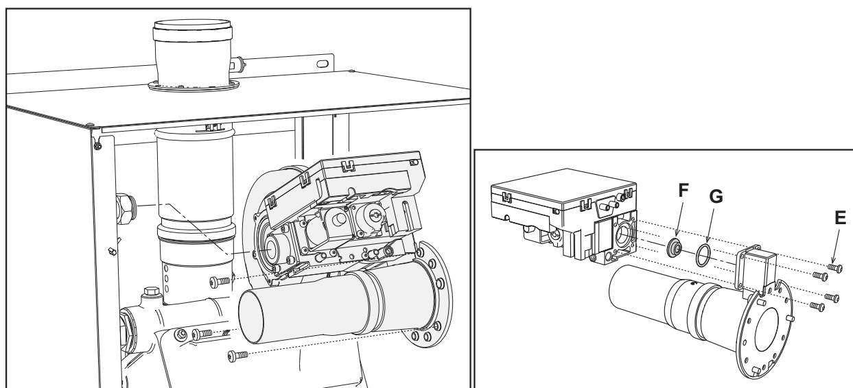
wygląd 58- Modele FORCE W 99, FORCE W 120 i FORCE W 150
