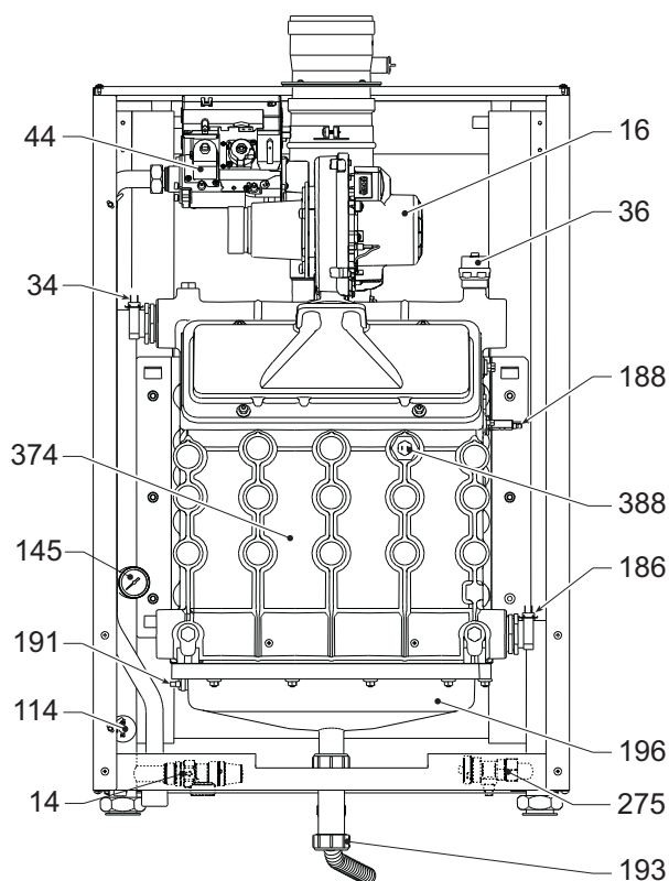
wygląd 70- Widok ogólny mod. FORCE W 150
