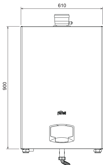
fig. 62- Vedere frontală
