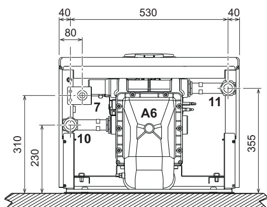
рис. 65- Вид снизу, мод. FORCE W 60 и FORCE W 80
