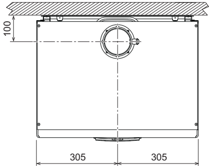
fig. 64- Vista superior
