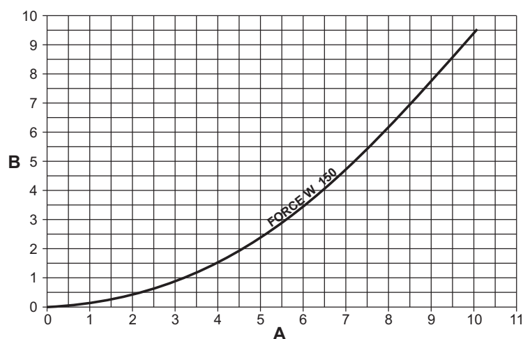
fig. 73- Diagramă pierderi de sarcină modelele FORCE W 150
