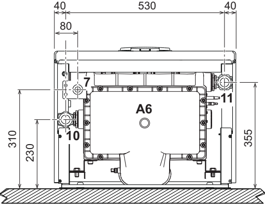
fig. 67- Vista inferior mod. FORCE W 150
