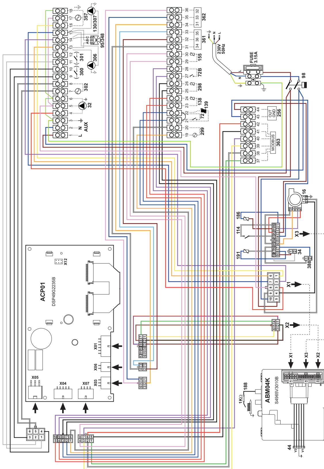
wygląd 74- Schemat elektryczny modeli FORCE W 60 oraz FORCE W 80
