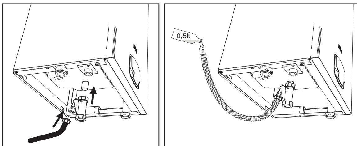
fig. 55- Racordarea evacuării condensului
