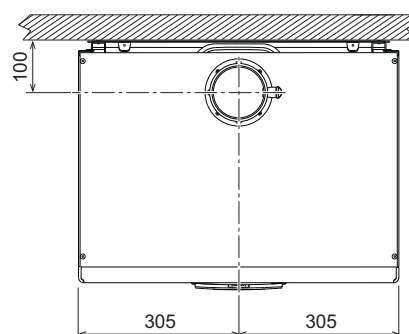
рис. 64- Вид сверху
