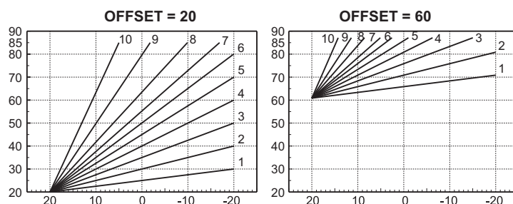
wygląd 30- Przykład przesunięcia równoległego krzywych kompensacji
