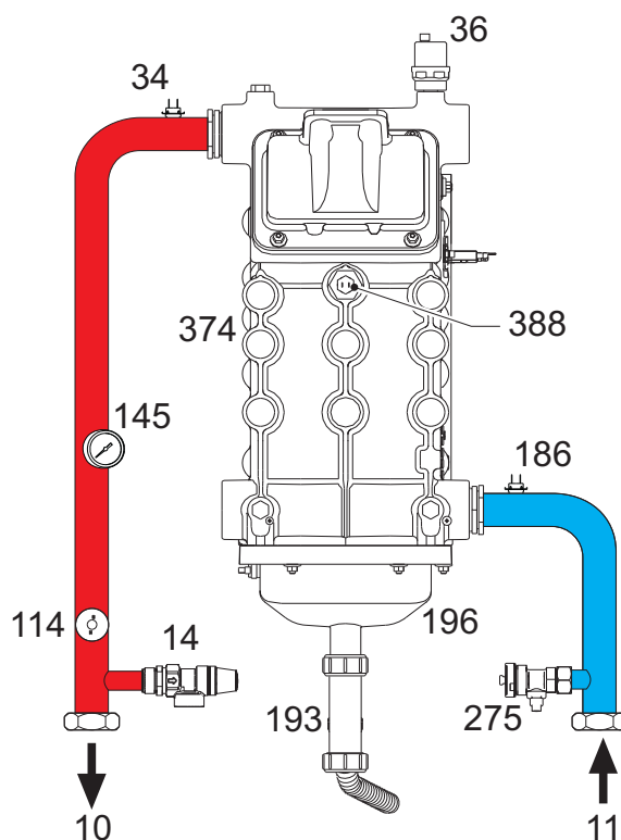
fig. 71- Circuitul hidraulic
