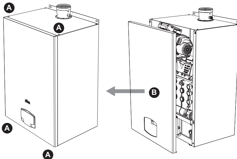
wygląd 61- Otwarcie panelu przedniego
