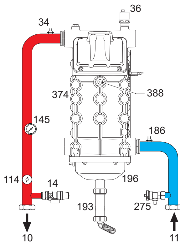
fig. 71 - Circuito idraulico
