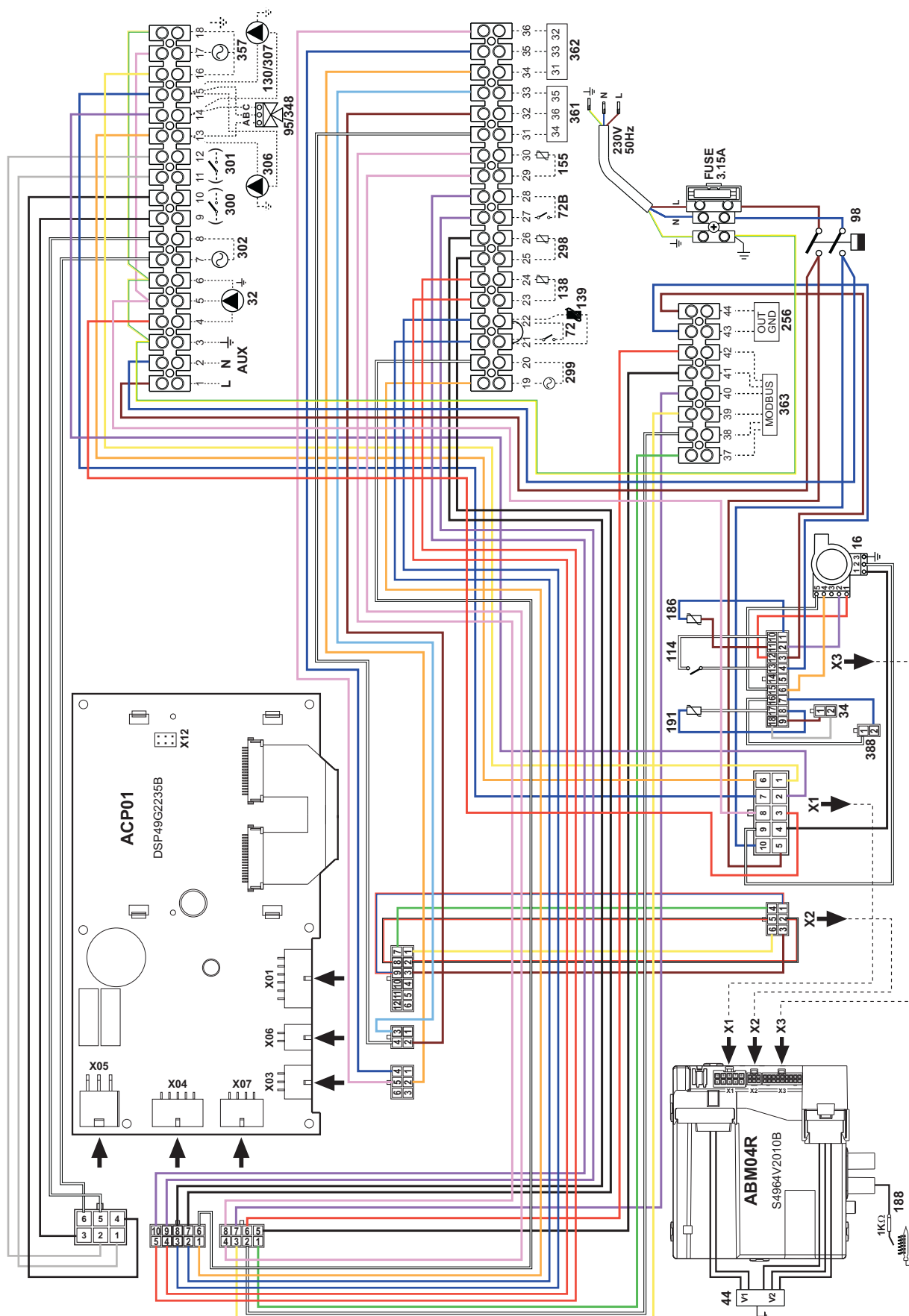
рис. 75- Электрическая схема моделей FORCE W 99, FORCE W 120 и FORCE W 150
