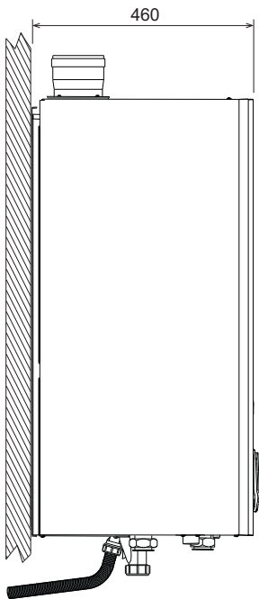
fig. 63- Vista lateral
