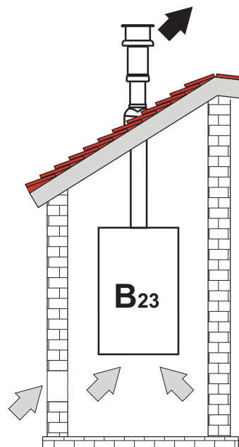
fig. 54- Ejemplos de conexión (⇨ = aire / ⇨ = humos)
