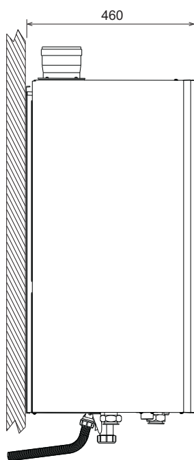
fig. 63 - Vista laterale
