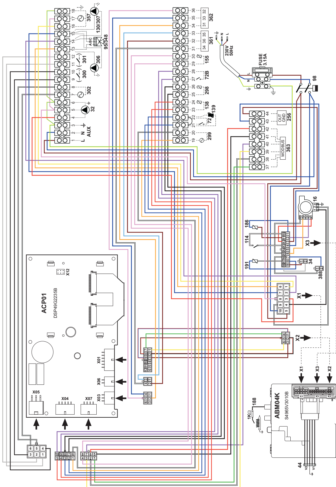
fig. 74- Schemă electrică modelele FORCE W 60 și FORCE W 80
