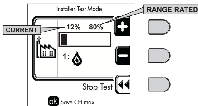
fig. 59- Modul TEST (exemplu putere de încălzire = 80%)
