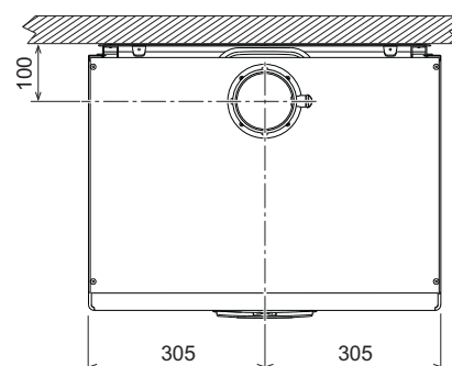
wygląd 64- Widok z góry
