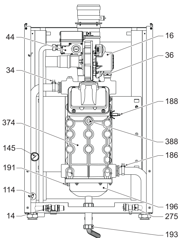
fig. 68- Vedere generală mod. FORCE W 60 și FORCE W 80
