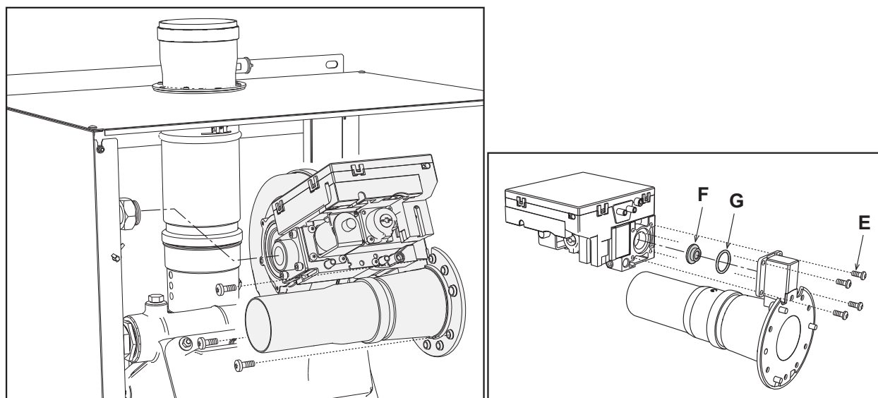
fig. 58- Modelele FORCE W 99, FORCE W 120 și FORCE W 150
