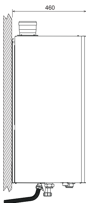
wygląd 63- Widok z boku
