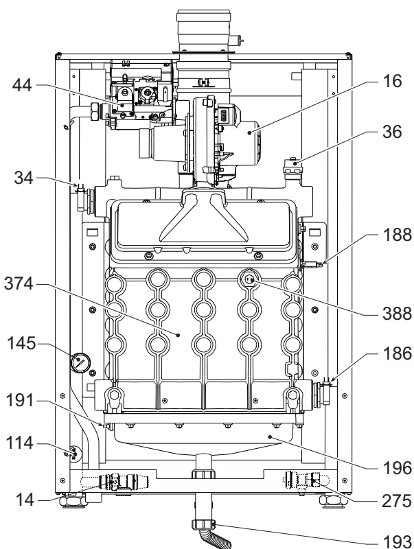
fig. 70 - Vista generale mod. FORCE W 150
