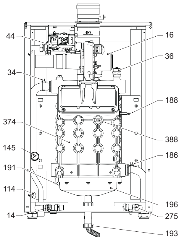
рис. 69- Общий вид, мод. FORCE W 99 и FORCE W 120
