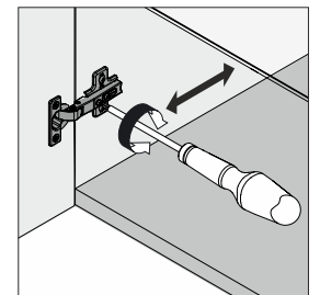
Regolazione dell'inclinazione Inclination adjustment Réglage de l'inclinaison
