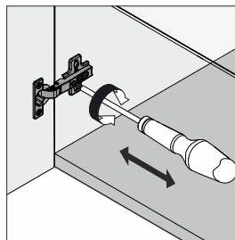
Regolazione laterale Lateral adjustment Réglage latéral
