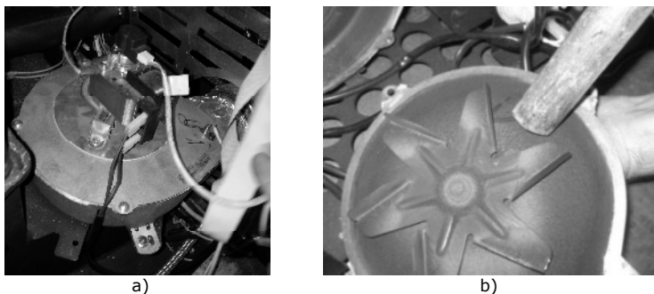
Figura 23 – a) Retirar os parafusos; b) Retirar o extractor
