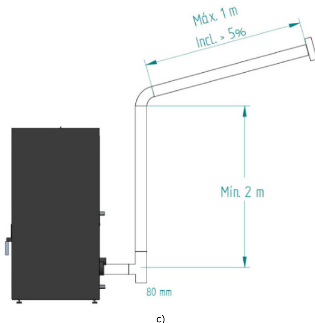
c) Figura 9 - Exemplos de instalações tipo
