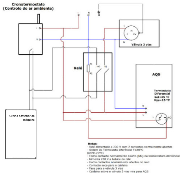
Figura 29 - Ligação eléctrica de um cronotermostato (controlo do ar ambiente) de um termostato diferencial ligado ao depósito de AQS e da válvula de três vias a uma caixa de relés
