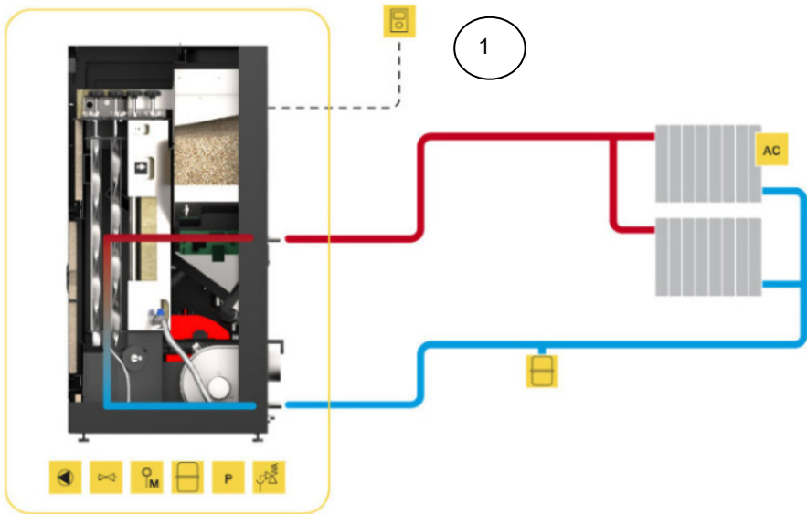
Figura 27 - Com ligação simples apenas a radiadores de aquecimento central
