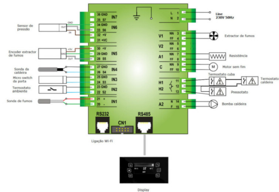
Figura 33 - Esquema eléctrico First Advance Hydro 13 kW
