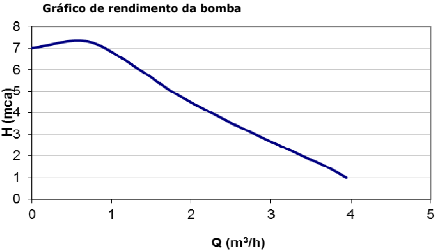
Figura 34 - Gráfico de desempenho da bomba
