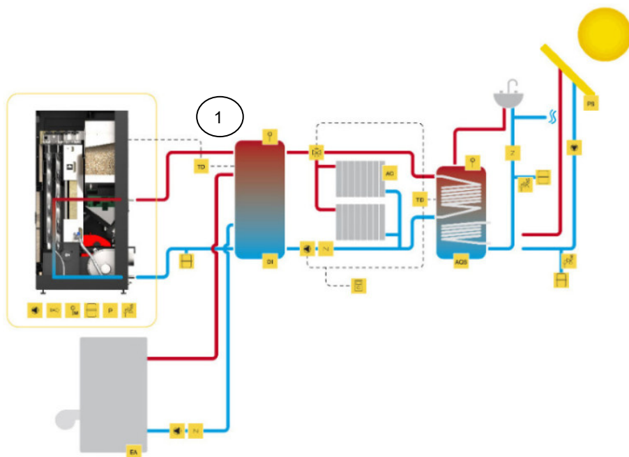
Figura 30 - Ligação a radiadores de aquecimento central, conjugado com outra salamandra de apoio e águas sanitárias combinado com painel solar
