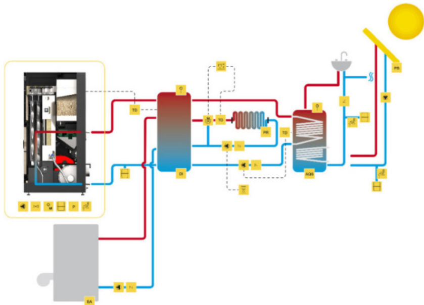
Figura 31 - Ligação a chão radiante, conjugado com outra salamandra de apoio e águas sanitárias combinado com painel solar
