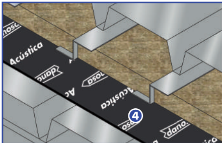
4 Cubiertas acústicas tipo deck (pegado a la chapa)
