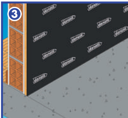
Fijar con fijaciones de aislamiento.
