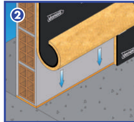
Presentar el producto con la parte amarilla a la pared.
