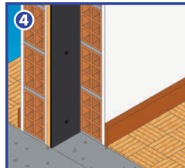
Construir el 2º tabique.
