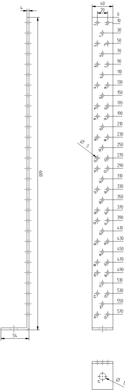
Figure A.85 hold-down 8799 6004 1E
