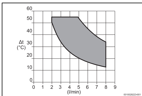
Fig. 29 Modelo 11 litros
