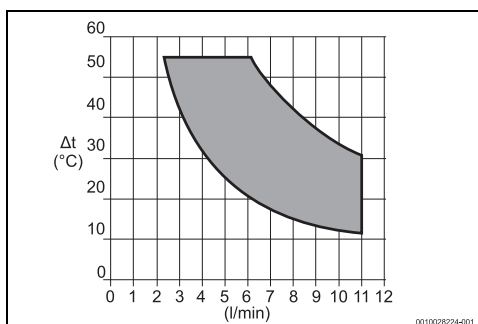
Fig. 30 Modelo 14 litros
