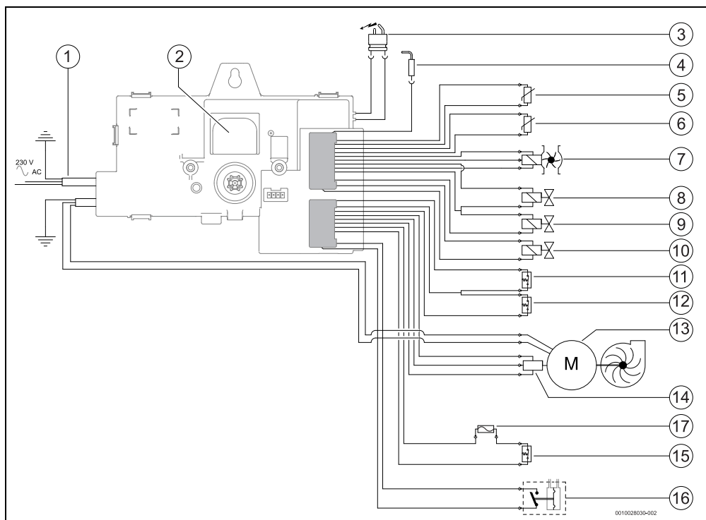
Fig. 28 Esquema eléctrico
