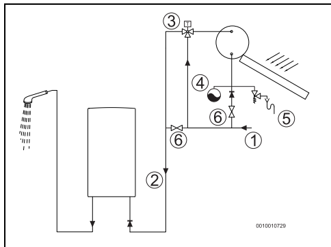
Fig. 14 Instalação solar
