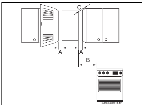
Fig. 19 Distâncias mínimas
