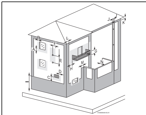
Fig. 20 Distâncias mínimas a pontos de exaustão
