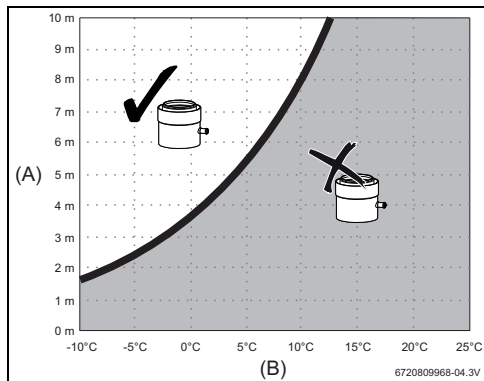
Fig. 16 Condutas concêntricas
