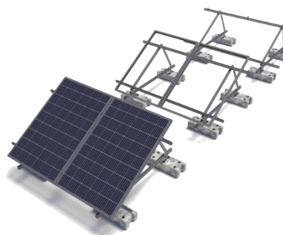
SOLSTAND™ fijación en contrapesos
