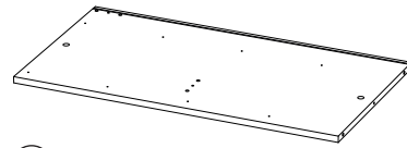
1 Costado derecho 839x460x16 Lateral Direito - Right side - Côte droit
