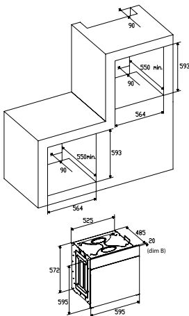
INBAUMAßE FÜR OFEN MIT TÜRDICKE 20 mm (dim B)
