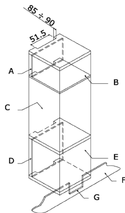
Fig. 8: Requisitos de ventilação e recorte para a instalação de um forno eléctrico simples num armário alto.
