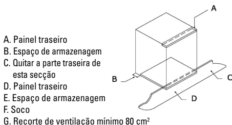
Fig. 7: Requisitos de ventilação e recorte para a instalação de um forno eléctrico simples numa unidade de cozinha standard. Requisitos de ventilação mínimos para as estantes superiores, de base e de suporte da parte traseira da unidade.
