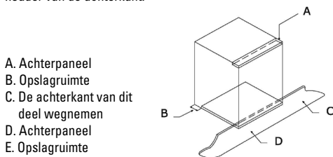
Fig. 7: Ventilatie- en afstandeisen voor de installatie van een eenvoudig elektrisch oven in een standaard keuken. Mindeste ventilatieeisen voor de bovenste rekken, bodem en houder van de achterkant.
