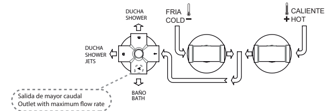
MODELOS BIMANDO + DISTRIBUIDOR 3 VIAS 2 HANDLE MODEL + 3 WAY DIVERTER
