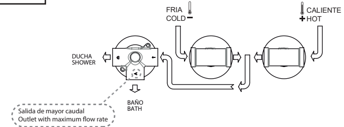
MODELOS BIMANDO + DISTRIBUIDOR 2 VIAS 2 HANDLE MODEL + 2 WAY DIVERTER
