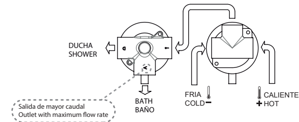
MODELOS MONOMANDO + DISTRIBUIDOR 2 VIAS SINGLE LEVER MODEL + 2 WAY DIVERTER
