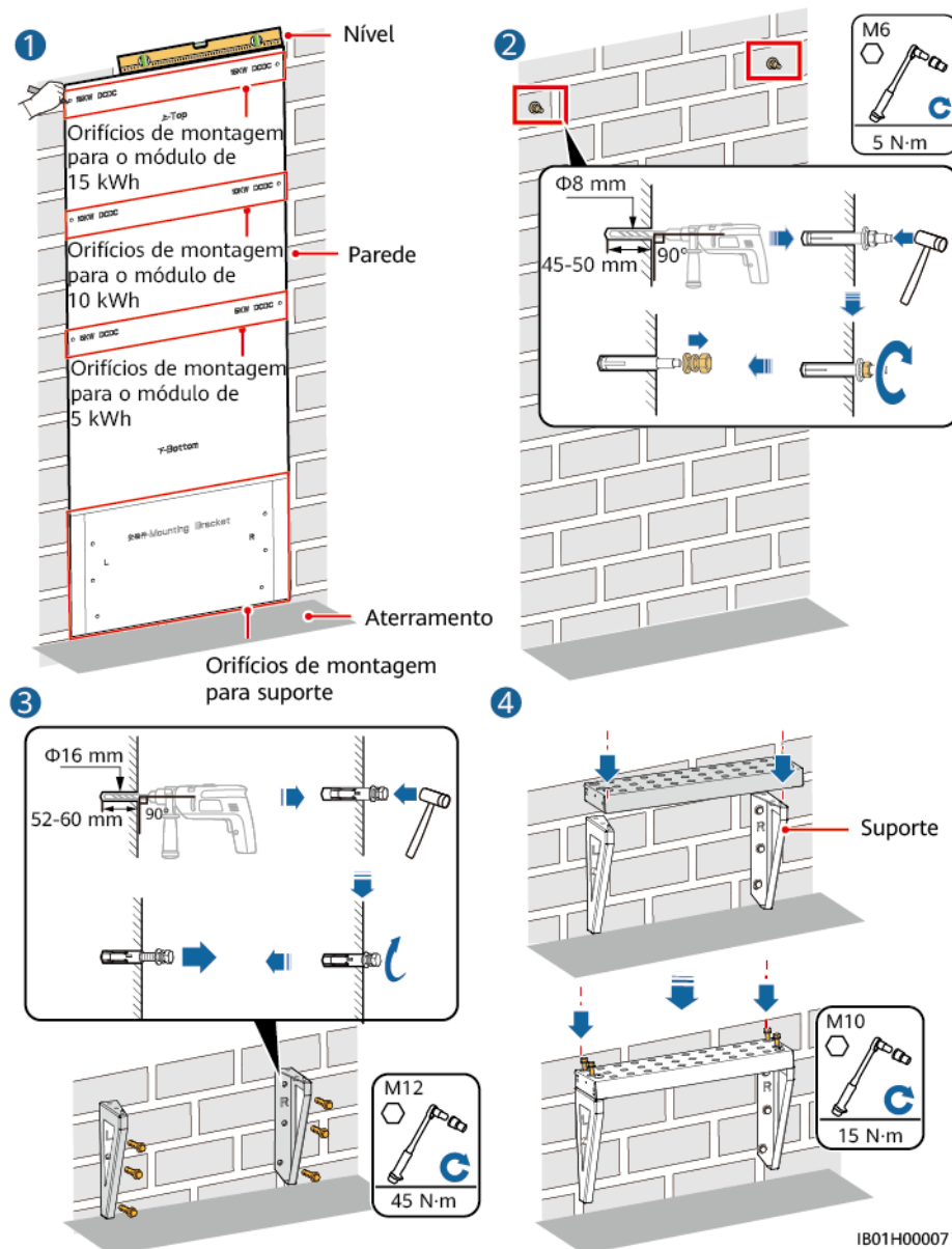
Figura 4-8 Montagem na parede
