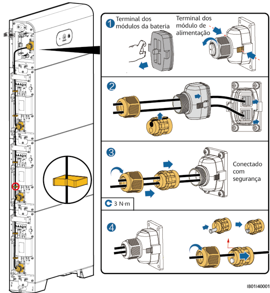
Figura 5-4 Conexões do cabo de sinal entre o módulo de alimentação e os módulos da bateria
