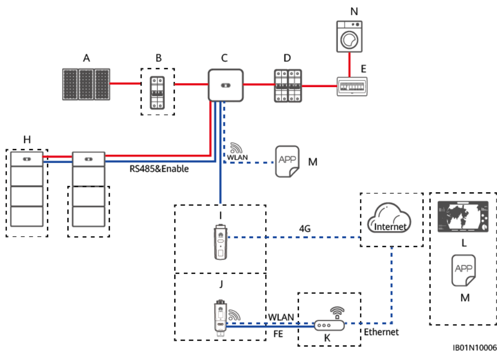
Figura 3-13 ESS não conectado à rede elétrica (caixas tracejadas indicam componentes opcionais)
