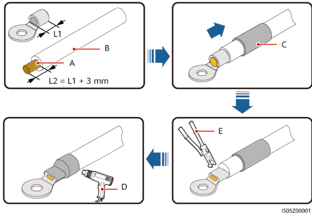
Figura 5-6 Crimpagem de um terminal OT
