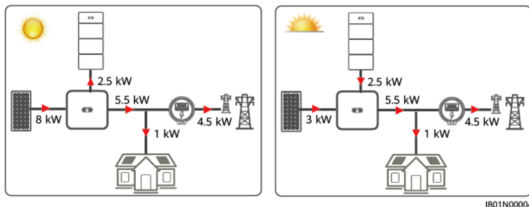
Figura 3-8 Exemplo de Totalmente fornecida à rede
