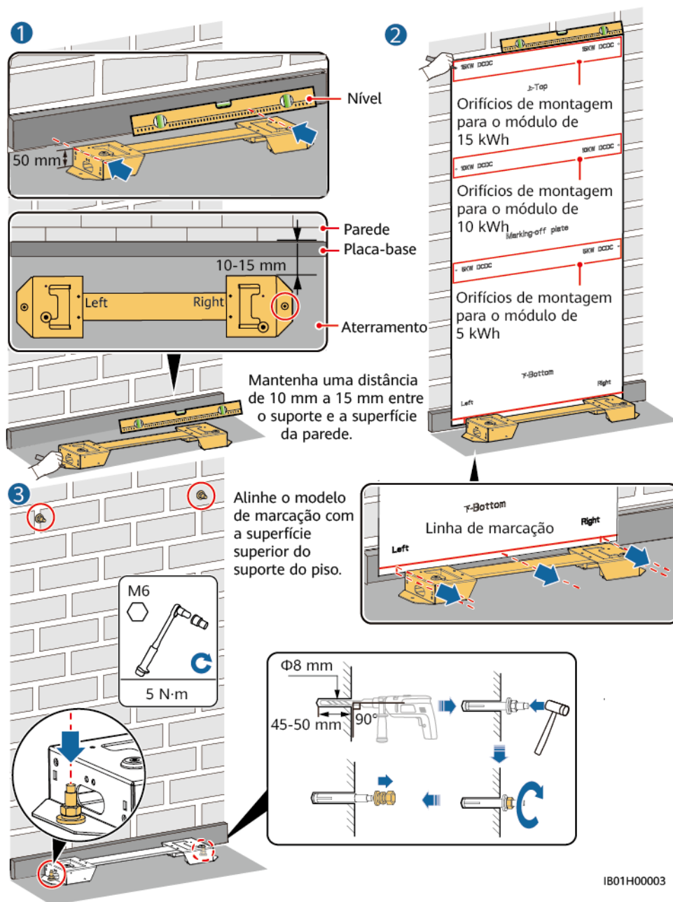
Figura 4-4 Instalação dos parafusos de expansão
