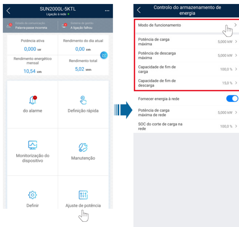
Figura 3-4 Configuração do parâmetro de controle da bateria
