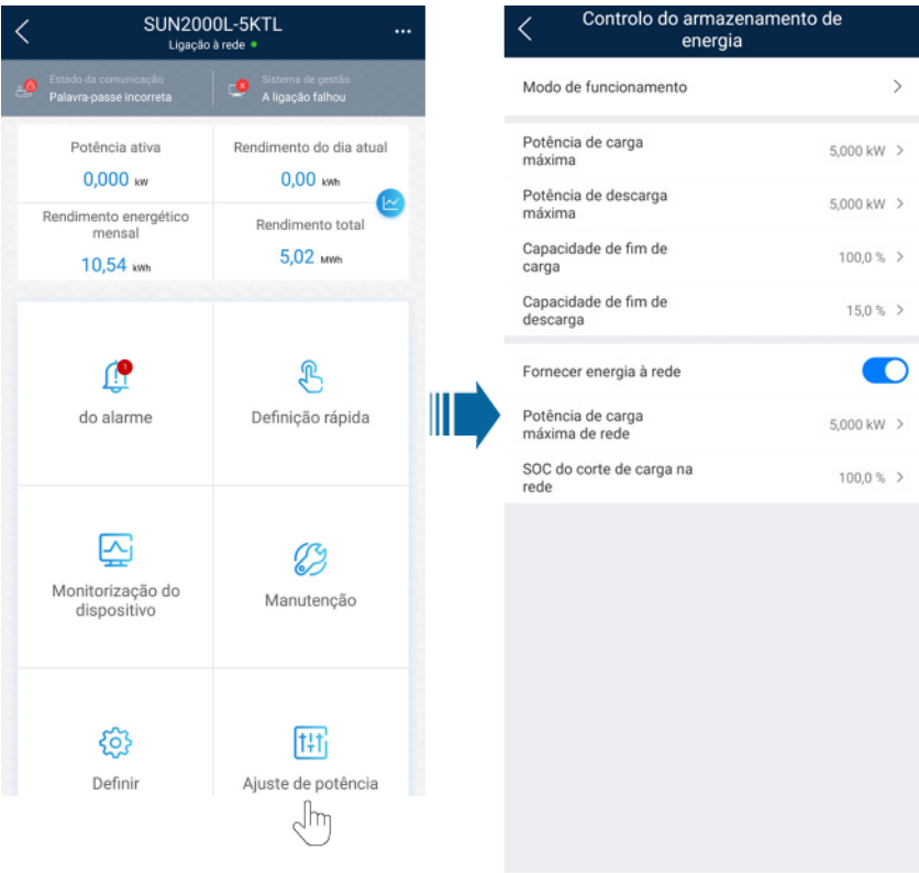
Figura 6-4 Configuração do parâmetro de controle da bateria
