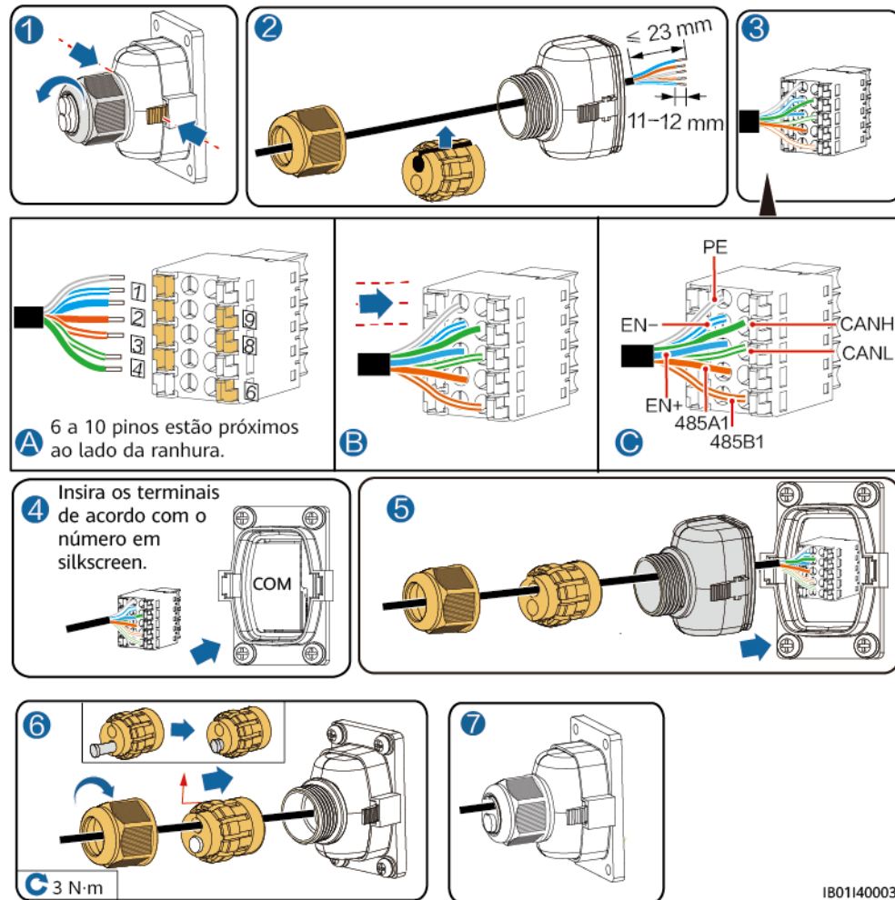
Figura 5-15 Terminal de comunicação em cascata
