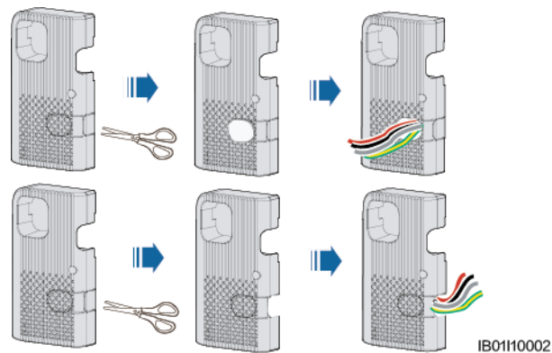
Figura 5-5 Roteamento de cabos para fora do orifício do cabo
