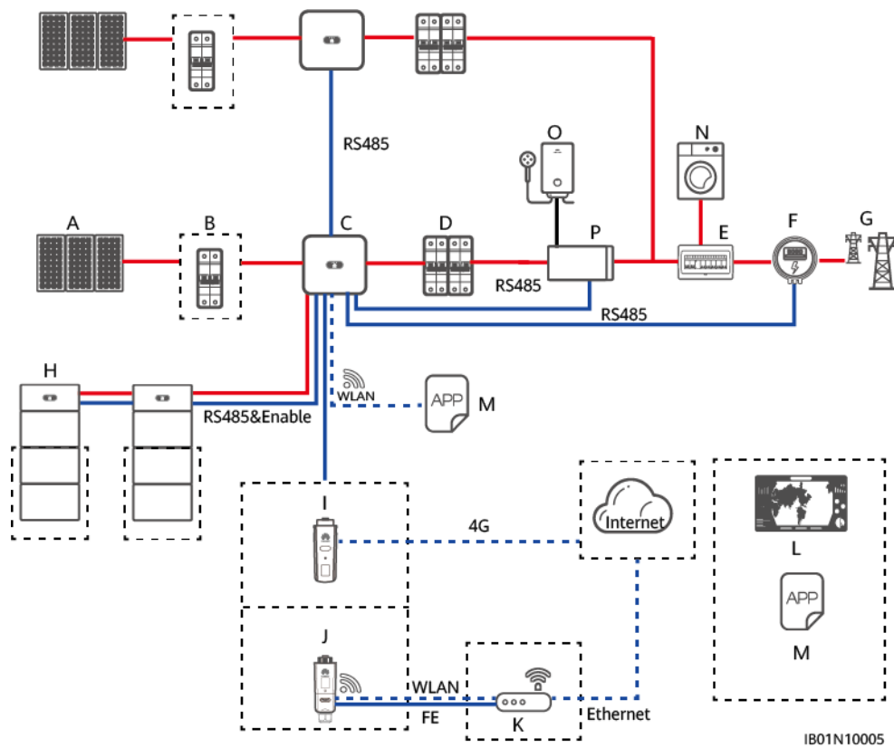
Figura 3-10 Inversor (com baterias) e inversor (sem baterias) (as caixas tracejadas indicam componentes opcionais)
