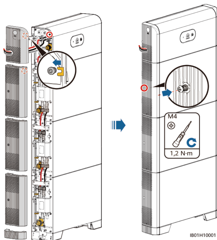
Figura 5-16 Instalação da tampa
