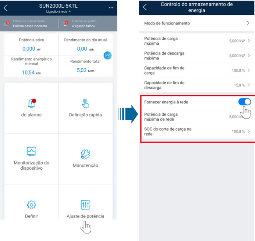
Figura 3-7 Configuração do parâmetro de controle da bateria
