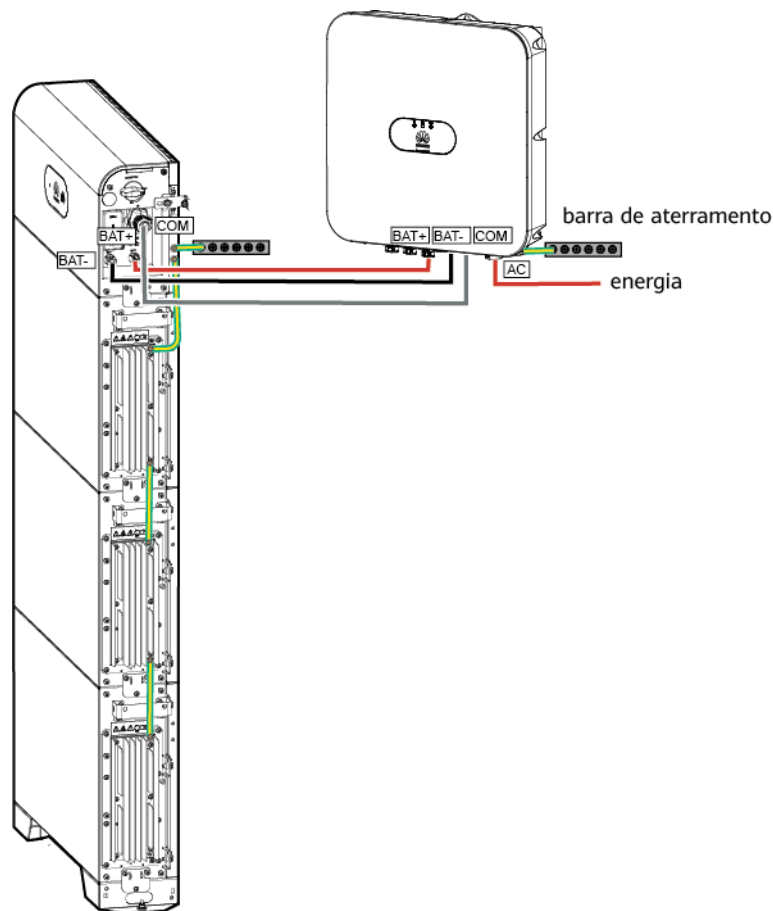
Figura 7-3 Diagrama de conexão do cabo
