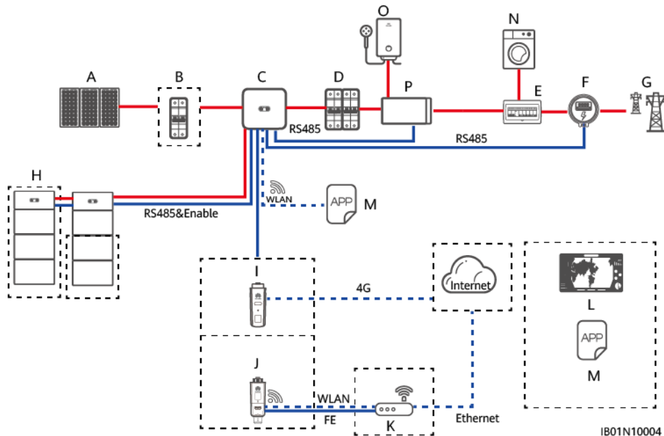
Figura 3-9 Rede ESS básica paralela não conectada à rede elétrica (caixas tracejadas indicam componentes opcionais)
