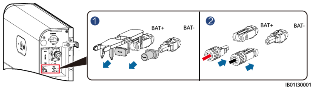
Figura 5-9 Conexão dos cabos da bateria
