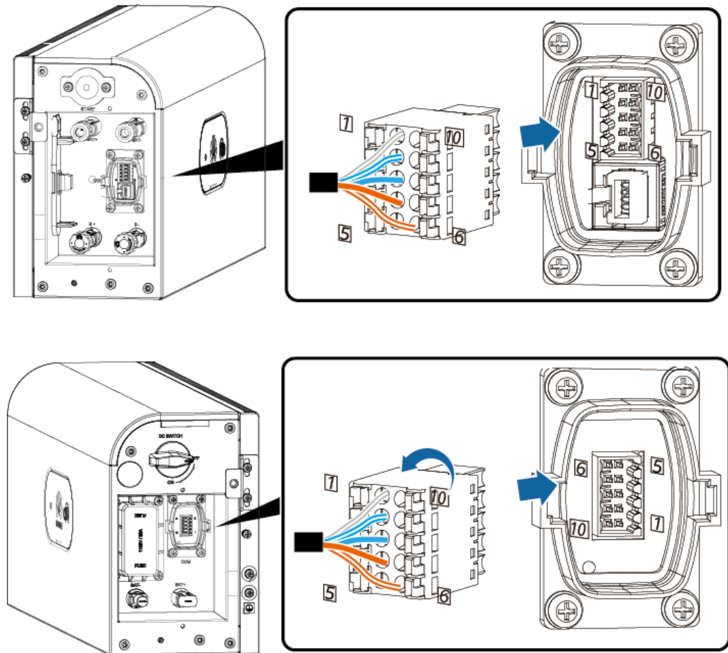
Figura 5-11 Inserção do terminal
