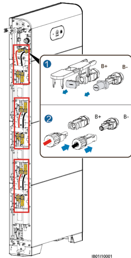
Figura 5-3 Conexão do cabo de alimentação CC dentro da bateria
