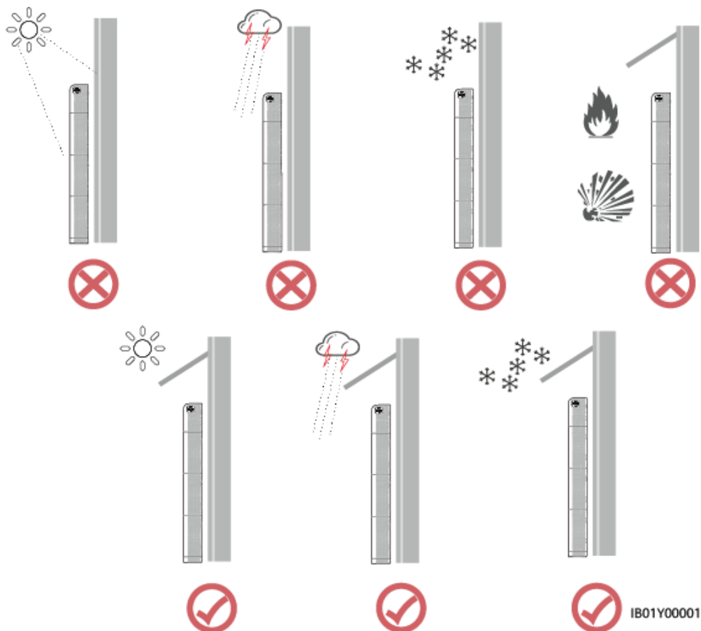
Figura 1-1 Ambiente de instalação
