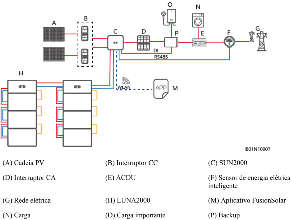
Figura 5-1 Conexões de cabo da bateria
