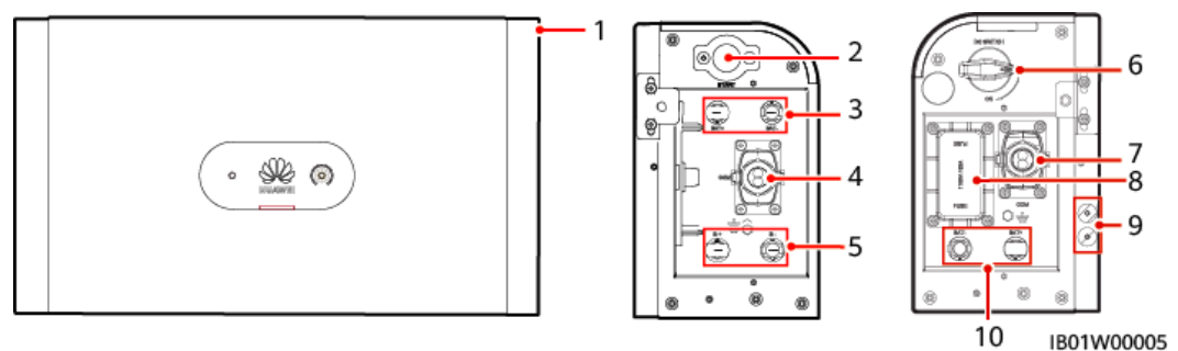
Figura 2-7 Módulo de controle de energia
