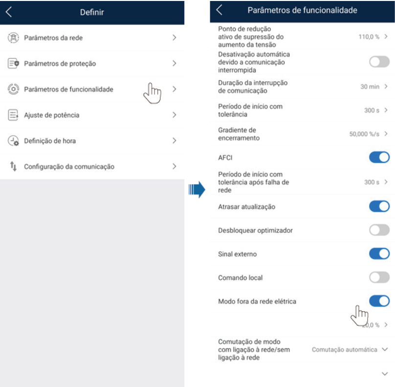
Figura 3-12 Configuração da energia de backup
