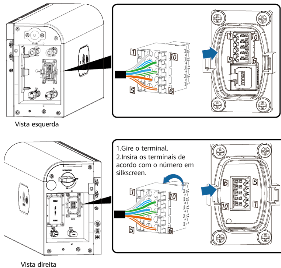
Figura 5-14 Inserção do terminal
