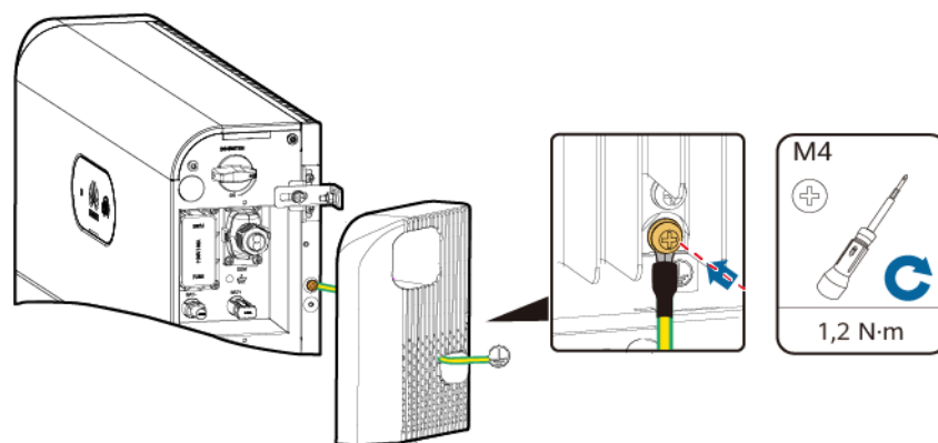
Figura 5-7 Aterramento do cabo PE
