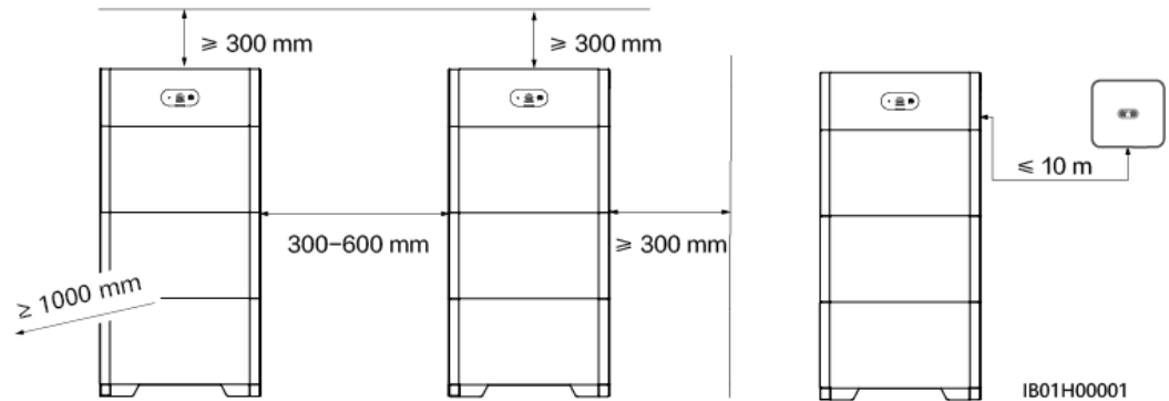
Figura 4-1 Espaço de instalação
