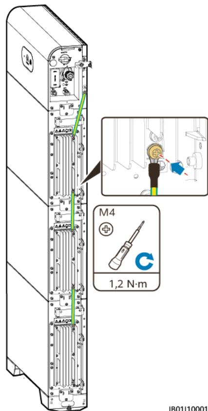
Figura 5-2 Conexão do cabo PE interno
