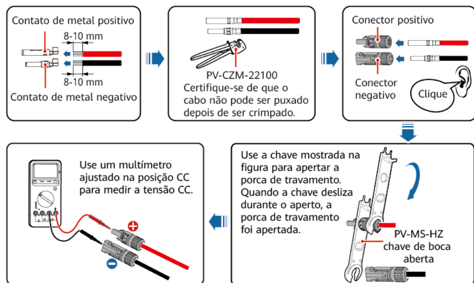
Figura 5-8 Montagem dos conectores CC
