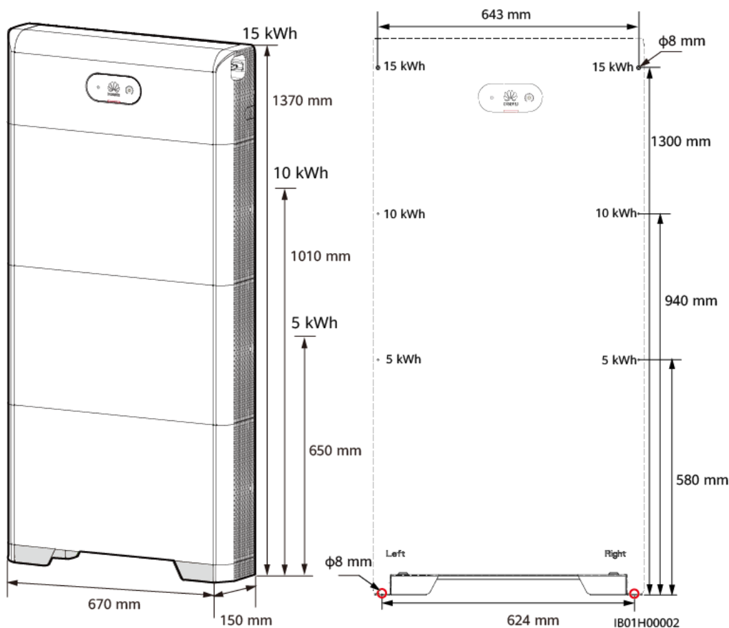
Figura 4-2 Dimensões da instalação no piso
