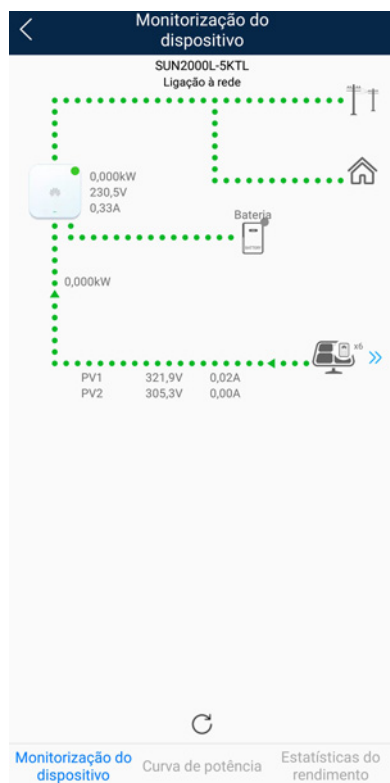
Figura 6-5 Monitorização do dispositivo
