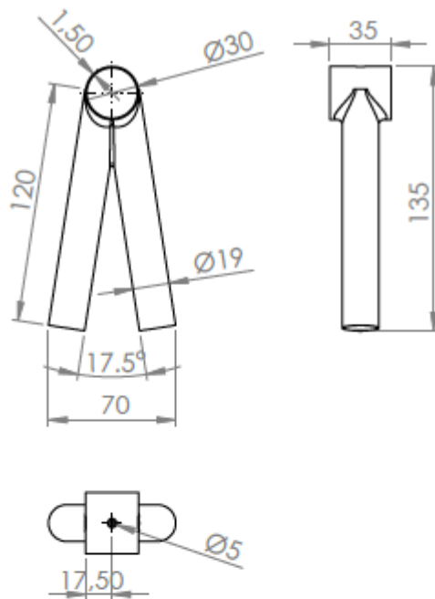
Bar Clip
