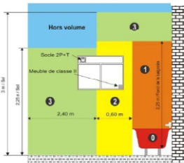
Graphique NFC 15-100/A5
