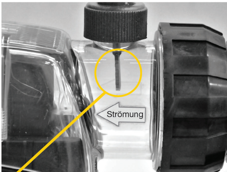
Abbildung B FEHLERHAFTER BETRIEB BEI LAUFENDER PUMPE
