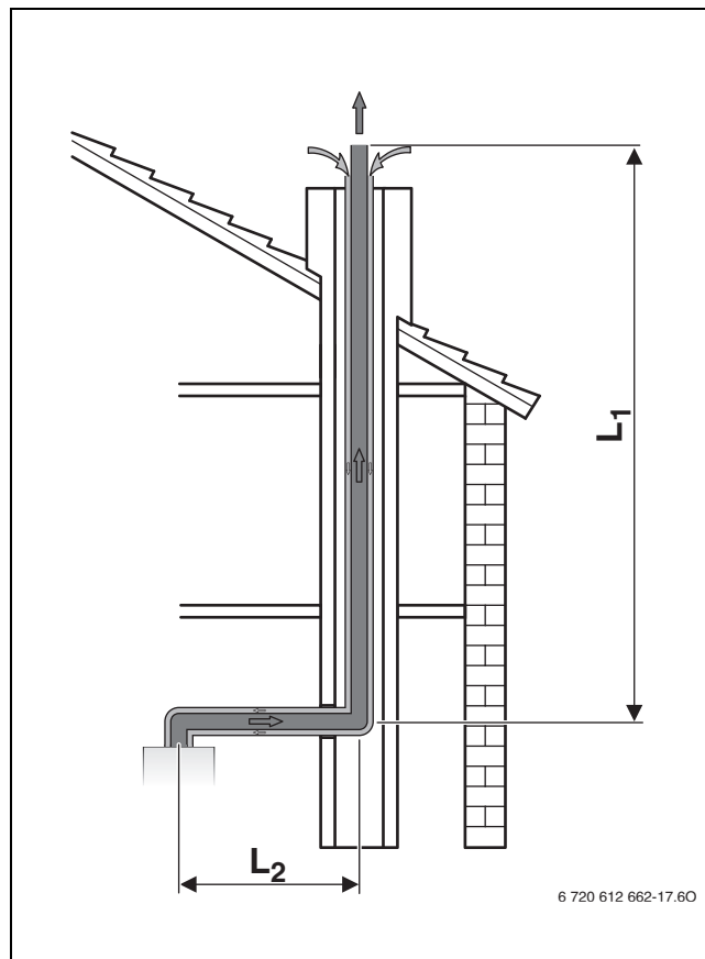
Fig. 9 Sistema di aspirazione aria/evacuazione dei prodotti della combustione con condotto concentrico nel camino secondo C 33
