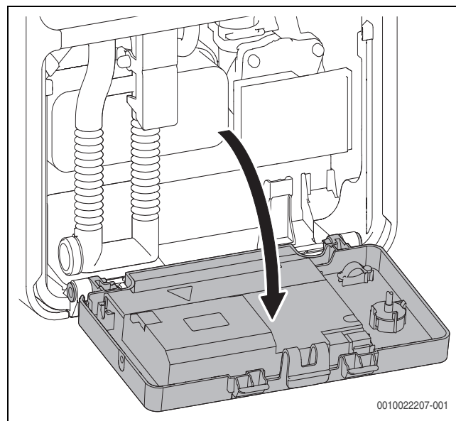
Fig. 28 Ribaltare verso il basso la scheda elettronica
