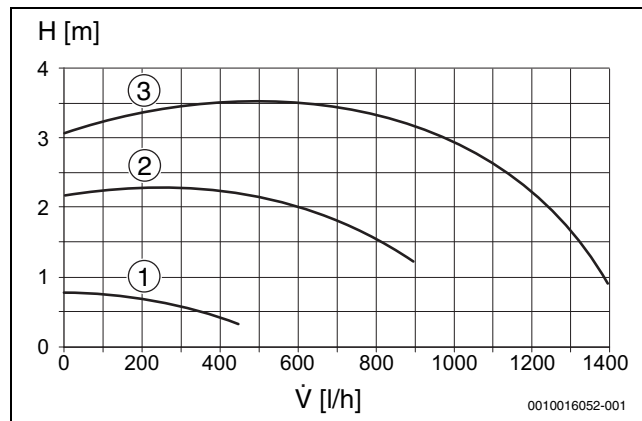
Fig. 36 Curva caratteristica del circolatore di riscaldamento (pressione proporzionale)
