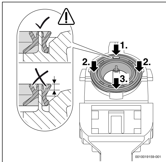
Fig. 56 Premere la guarnizione
