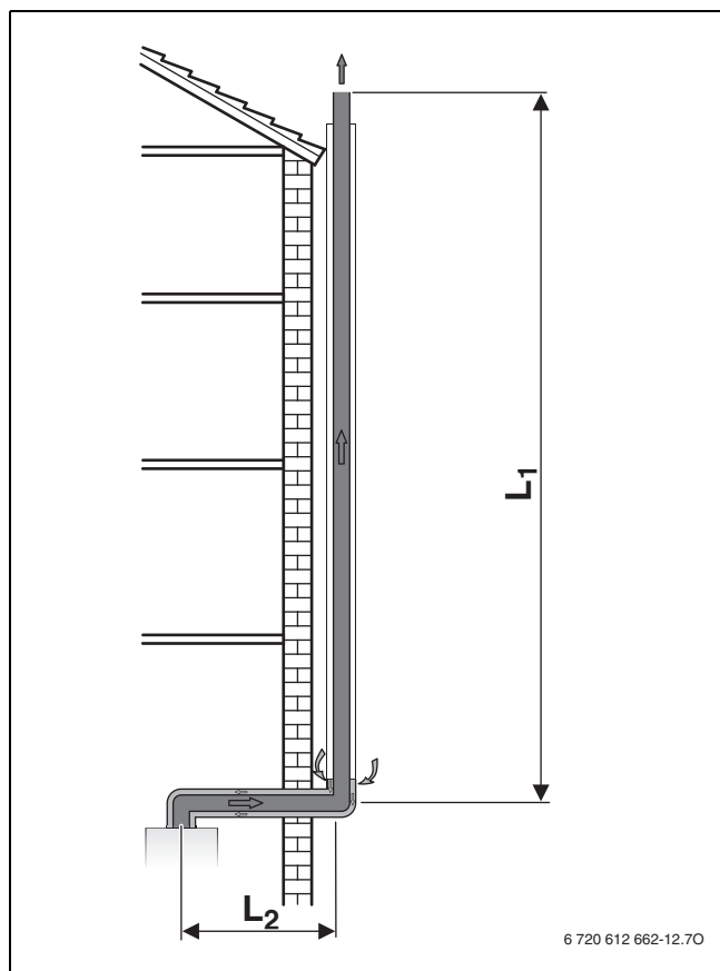
Fig. 16 Passaggio gas combusti sulla facciata secondo C 53
