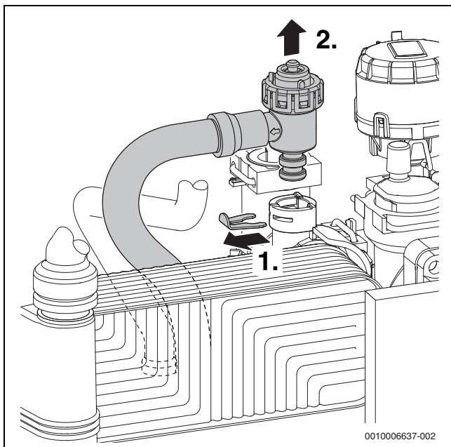
Fig. 58 Rimozione della valvola di sicurezza (circuito di riscaldamento)
