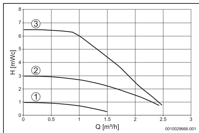
Fig. 35 Curva caratteristica del circolatore di riscaldamento (pressione costante)
