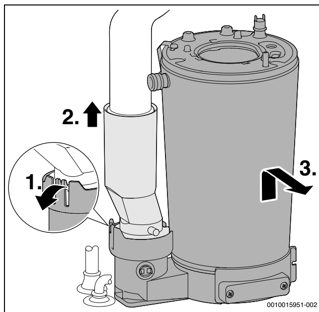
Fig. 67 Smontaggio dello scambiatore primario
