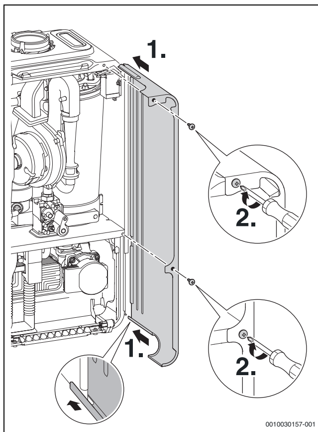
Fig. 70 Applicazione del rivestimento laterale
