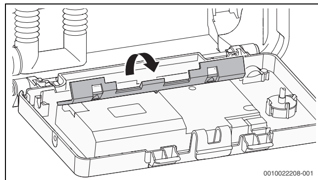
Fig. 29 Aprire la copertura
