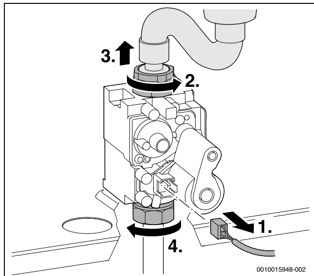
Fig. 61 Estrarre il connettore e allentare i dadi di raccordo
