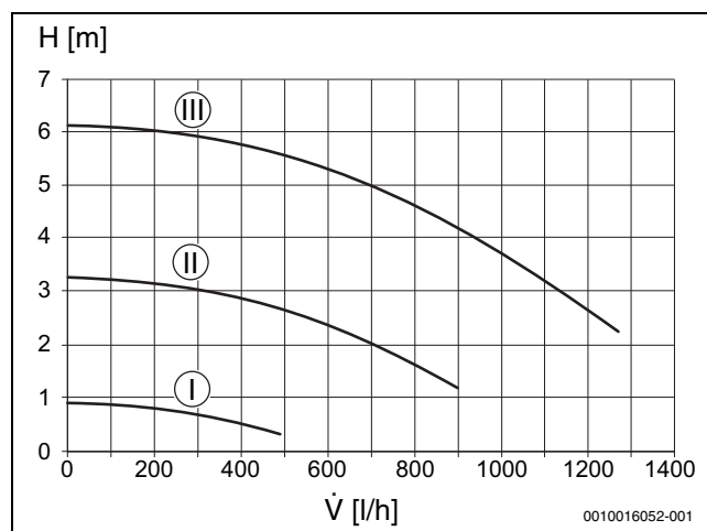
Fig. 34 Curva caratteristica del circolatore di riscaldamento (velocità costante)
