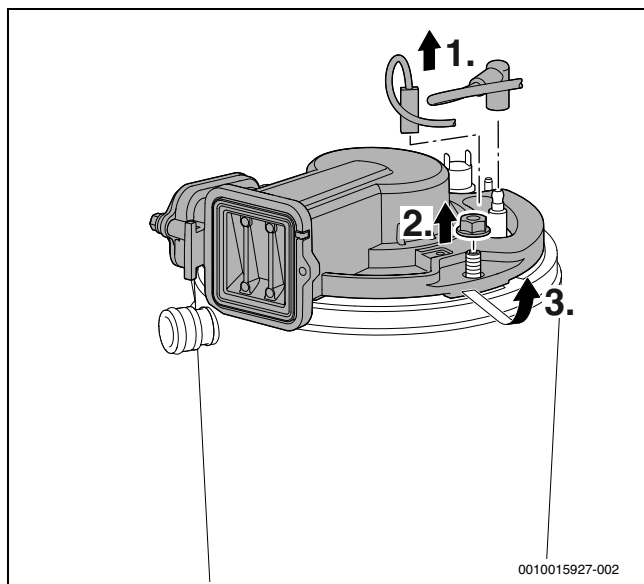
Fig. 44 Allentare il coperchio del bruciatore
