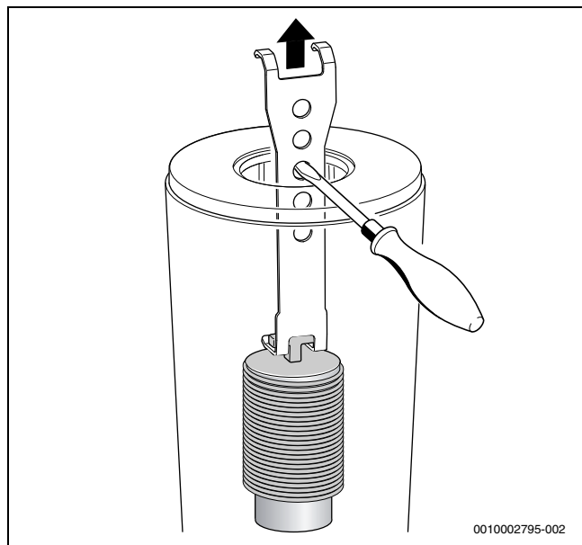
Fig. 48 Estrazione del deviatore di fiamma inferiore
