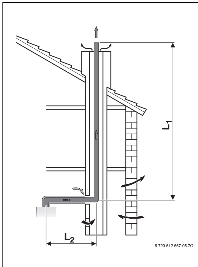
Fig. 8 Passaggio dei gas combusti nel camino secondo B 33
