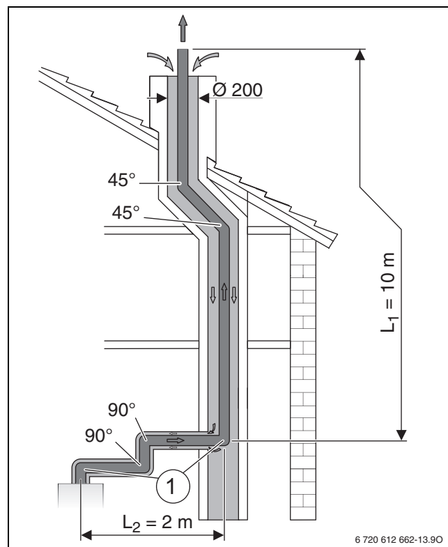
Fig. 17 Situazione di montaggio di un sistema di aspirazione aria/evacuazione dei prodotti della combustione nel camino secondo C_{93}
