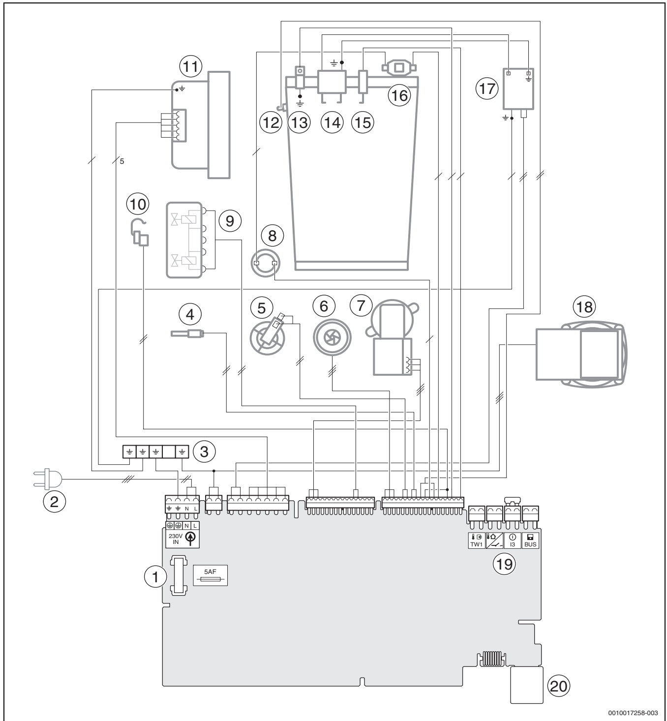
Fig. 73 Cablaggio elettrico
