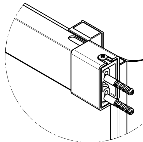
Dettaglio G Scala: 1:2
