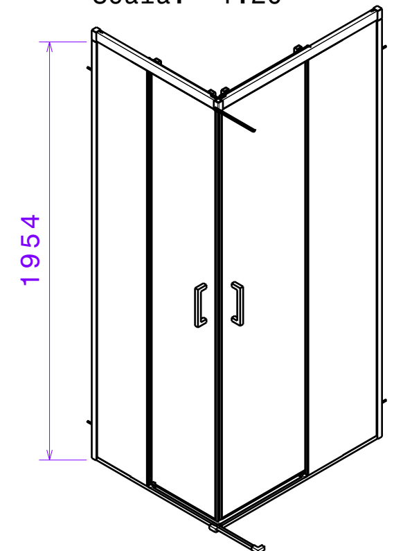
Vista isometrica Scala: 1:20
