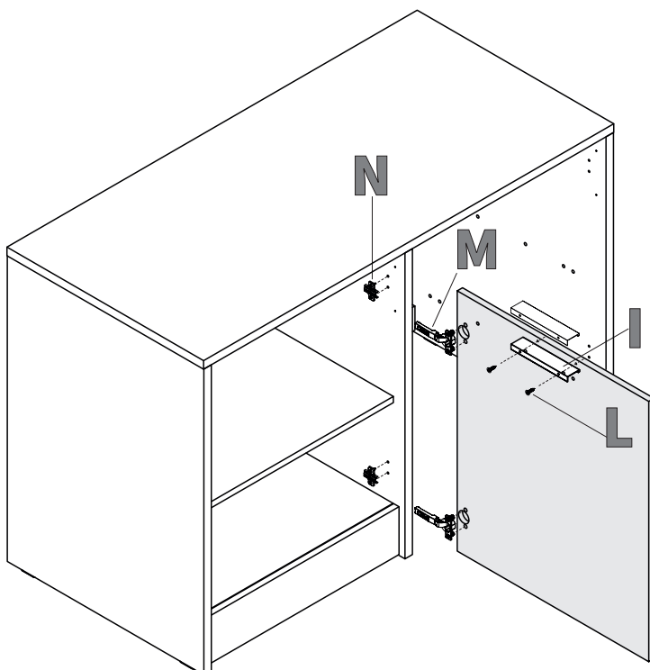
IT-Montaggio anta dx /EN- Door assembly rh/FR-Montage de porte dr
