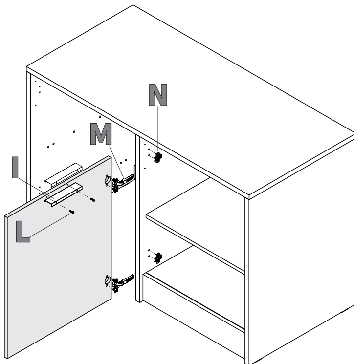
IT-Montaggio anta sx /EN- Door assembly lh/FR-Montage de porte gh
