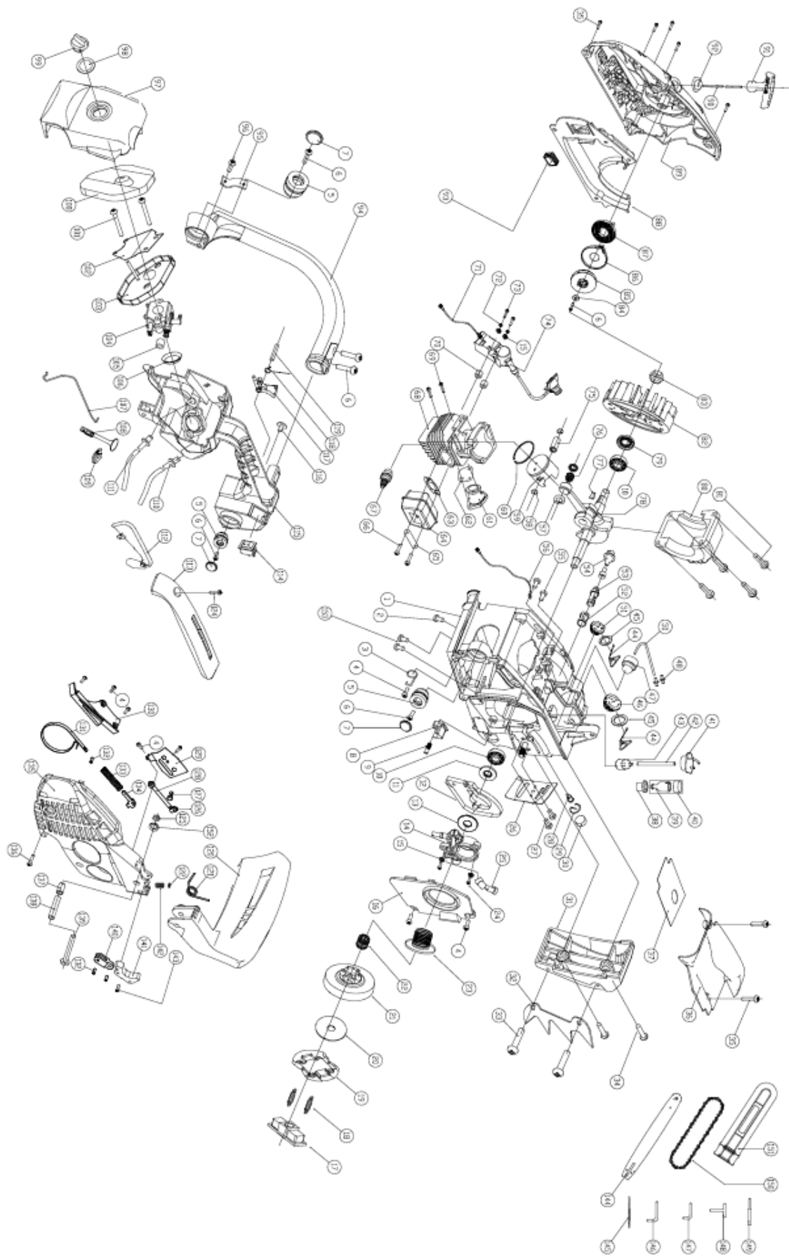
RYSUNEK ZŁOŻENIOWY Lider RG2600-12
