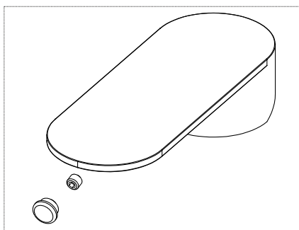
Leva
