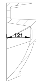
SEZIONE B-B
