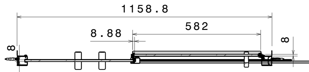
Vista in sezione A-A Scala: 1:10
