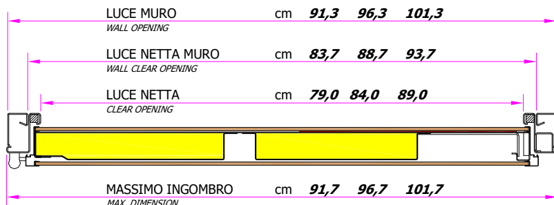
- SEZIONE ORIZZONTALE - HORIZONTAL SECTION
