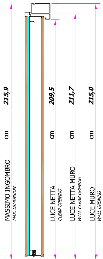
- SEZIONE VERTICALE - VERTICAL SECTION
