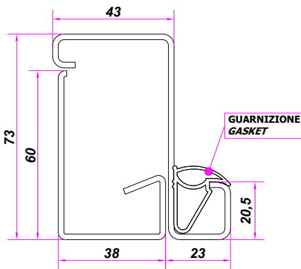
CONTROTELAIO E TELAIO SUBFRAME AND FRAME
