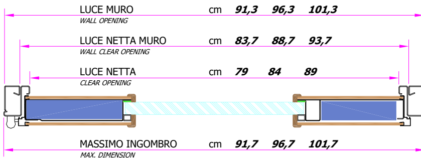
- SEZIONE ORIZZONTALE - HORIZONTAL SECTION
