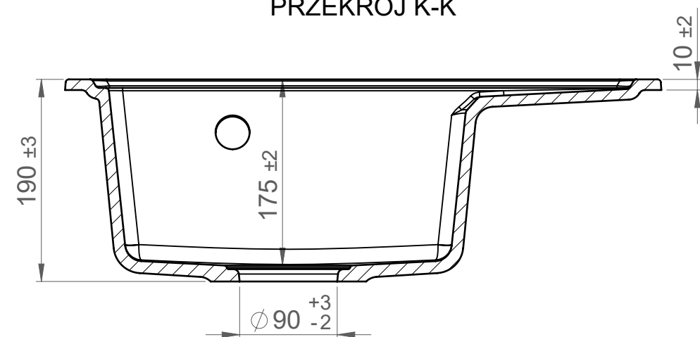
PRZEKRÓJ K-K
