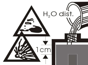
Figura 2: verifique el nivel de ácido de la batería. Añada agua destilada si necesario.
