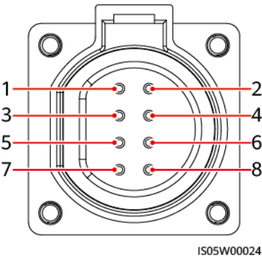
Figura 5-18 Portas dos cabos de sinal
