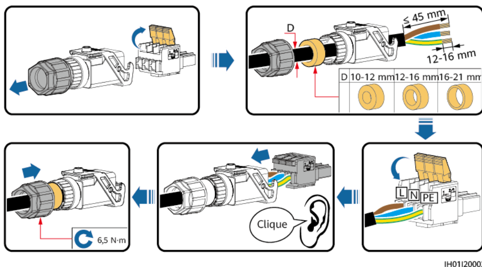
Figura 5-7 Montagem de um conector CA (três cabos condutores)
