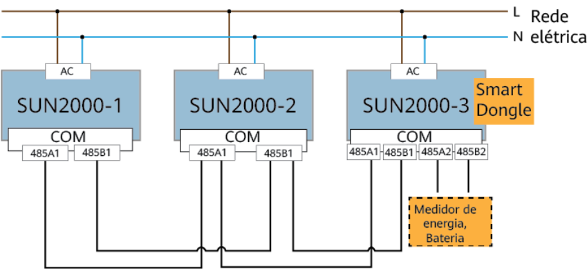
Figura 5-21 Ligação da rede elétrica em fase
