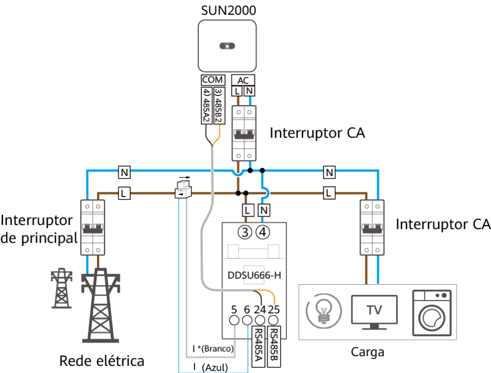
Figura 5-20 Ligação de cabos ao Smart Power Sensor (SUN2000 único)
