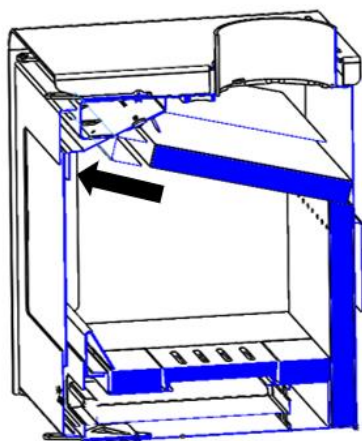
Figura nº10 - Primer movimiento para liberar el refuerzo
