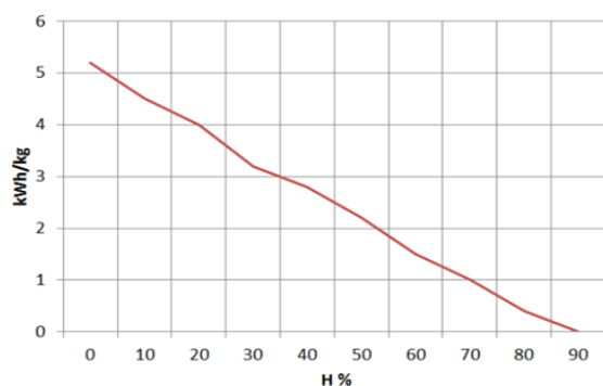
Figura nº6 - Relación entre humedad y poder calorífico de la leña.
