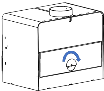
Figura nº8 - Registro de entrada aire doble combustión abierto
