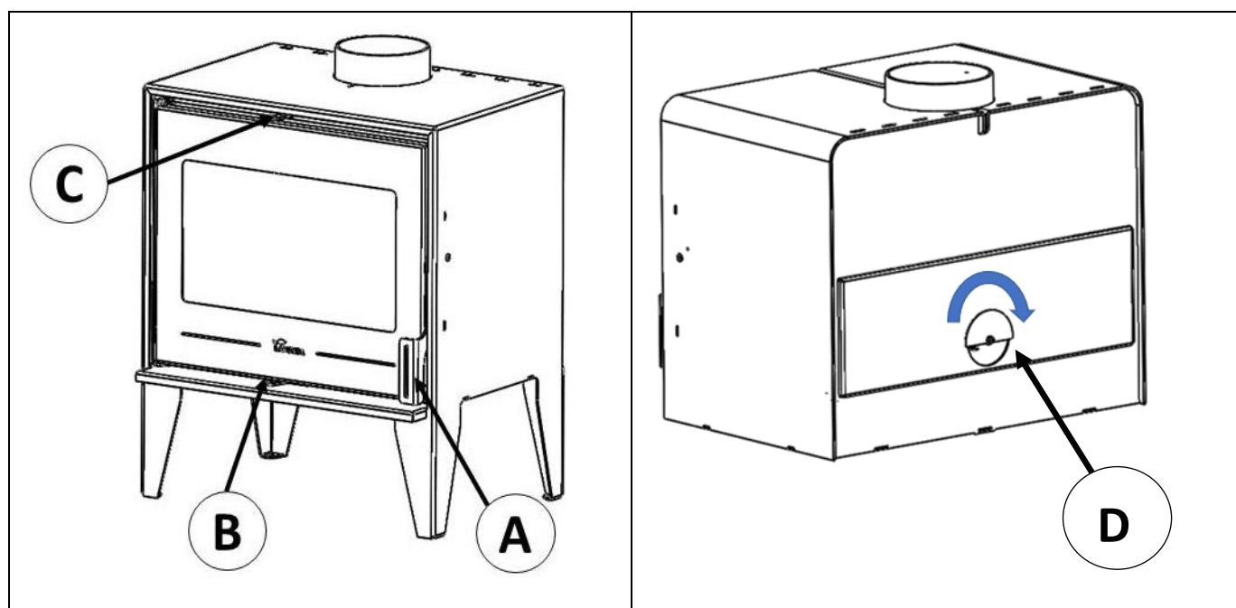
Figura nº7 - Elementos de funcionamiento del aparato
