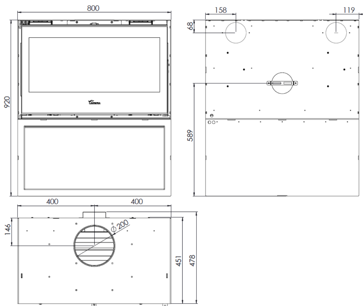
Figura nº2 - Dimensiones en mm del aparato ROCK 800 Plus
