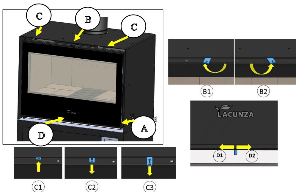
Figura n°13 - Elementos de funcionamiento del aparato
