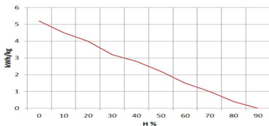
Figura n°12 - Relación entre humedad y poder calorífico de la leña.
