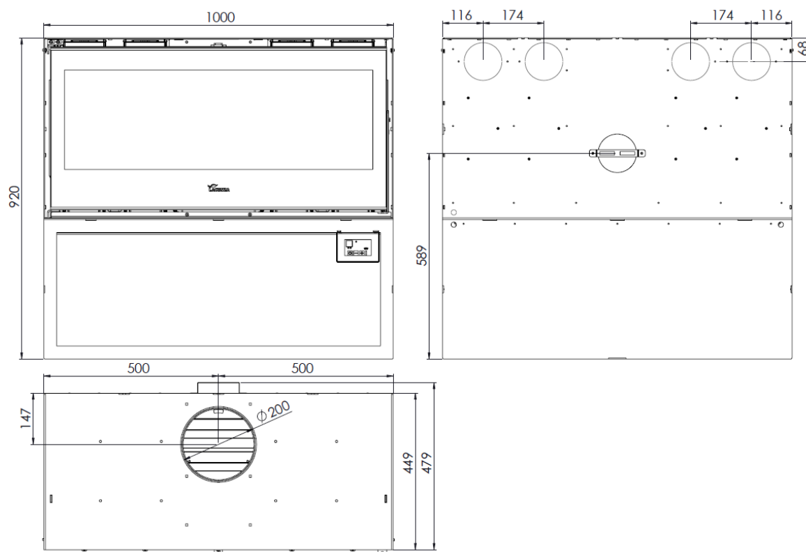
Figura nº3 - Dimensiones en mm del aparato ROCK 1000 Plus
