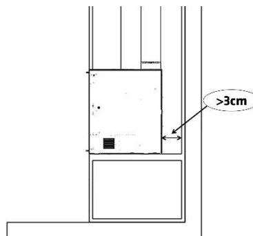
Figura nº7 - Separación entre el aparato y la pared trasera.
