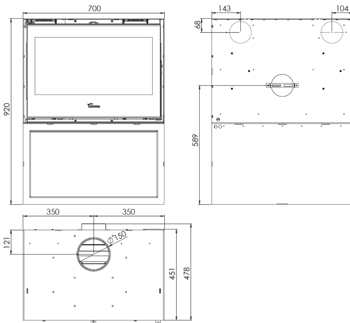
Figura nº1 - Dimensiones en mm del aparato ROCK 700 Plus
