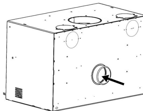
Figura nº8 - Entrada de aire conducida
