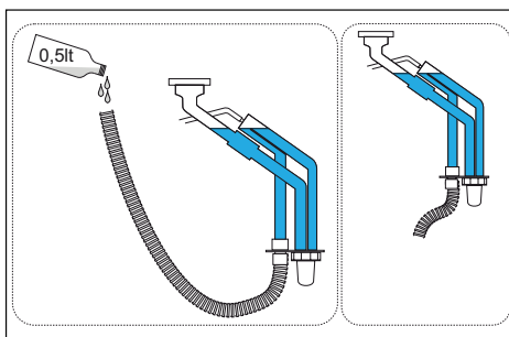
wygląd 28- Podłączenie spustu kondensatu
