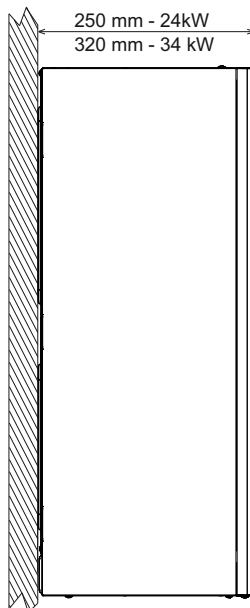
εικ. 33- Πλαϊνή όψη
