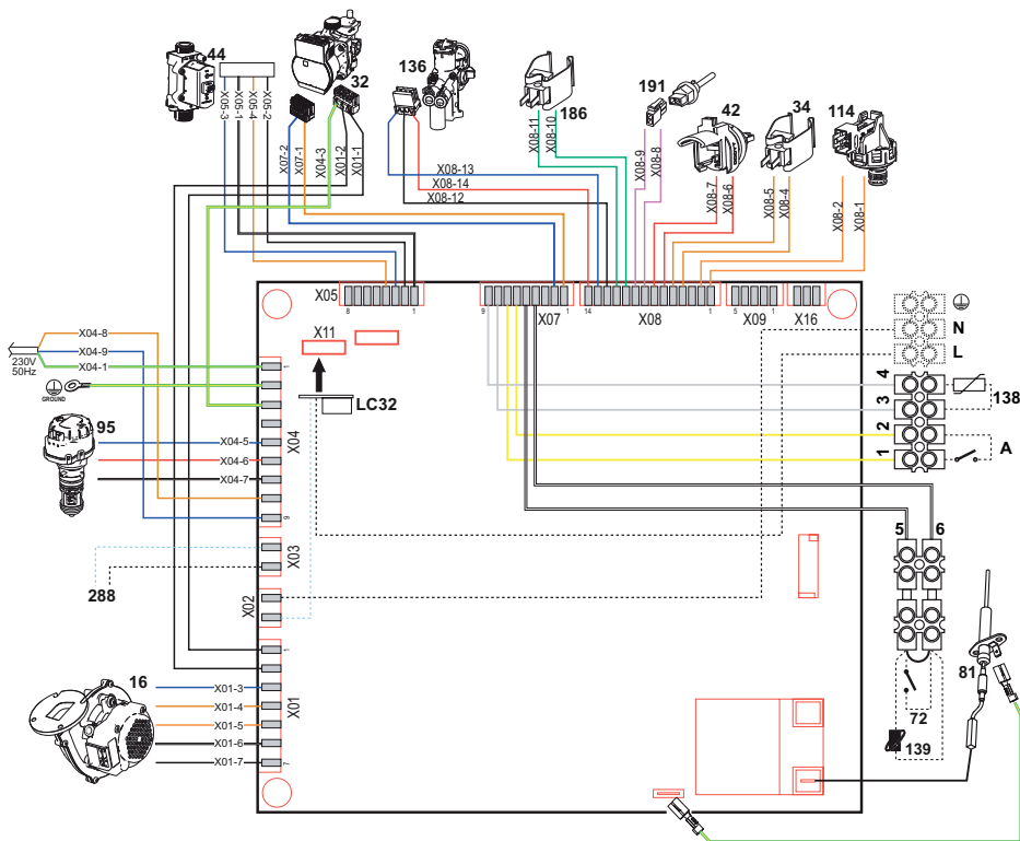
fig. 40 - Schema elettrico
