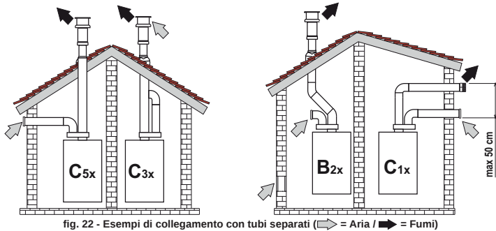
fig. 22 - Esempi di collegamento con tubi separati (⇨ = Aria / ⇨ = Fumi)
