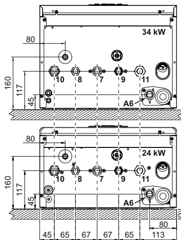
fig. 35 - Vista dal basso
