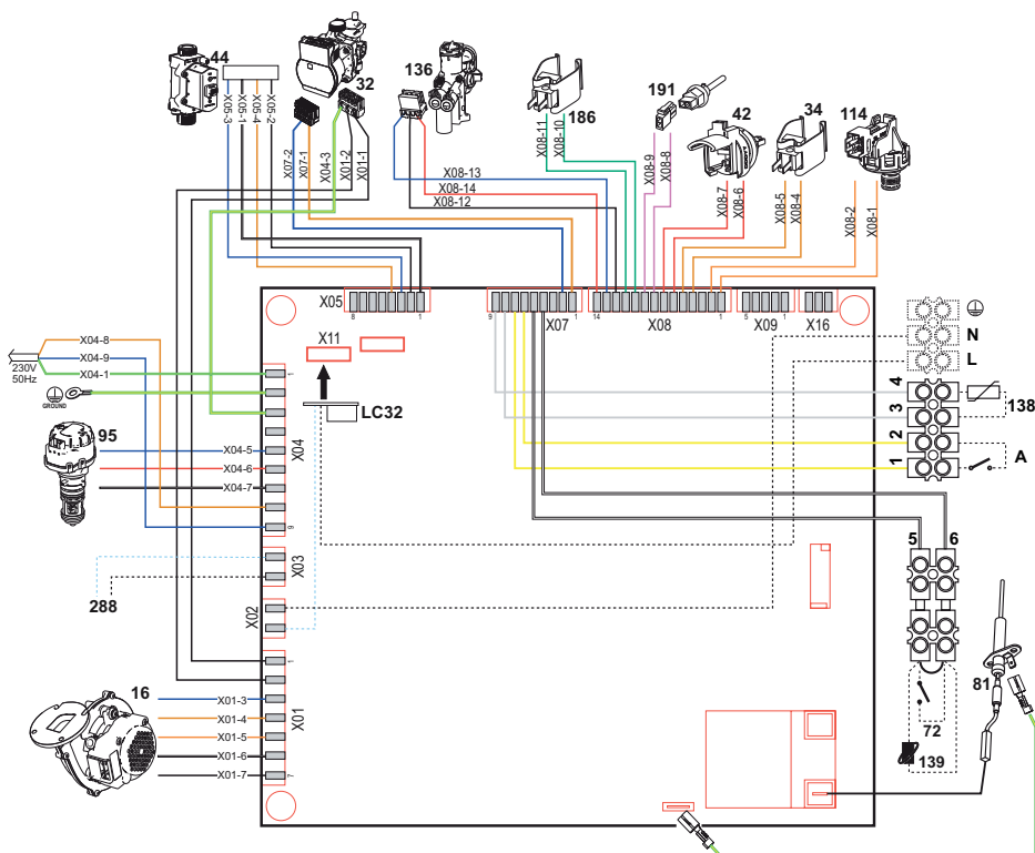
fig. 40- Schemă electrică
