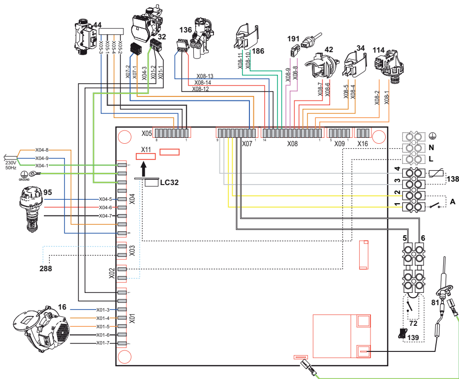
рис. 40- Электрическая схема
