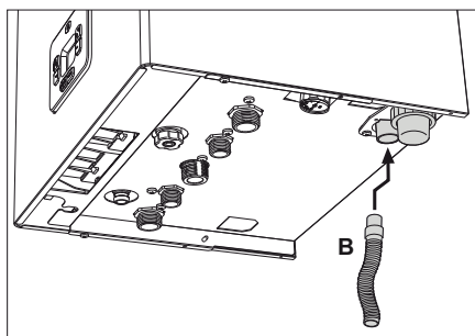
wygląd 28- Podłączenie spustu kondensatu
