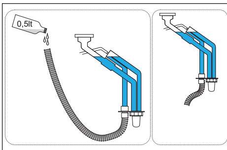
fig. 28- Racordarea evacuării condensului
