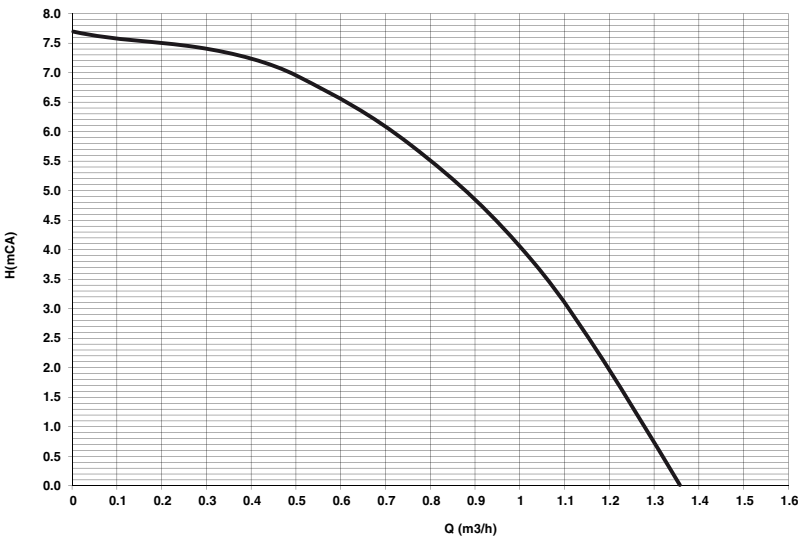
fig. 39 - Prevalenza residua disponibile all'impianto
