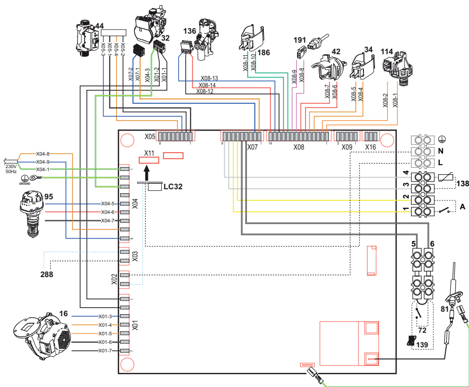
εικ. 40- Ηλεκτρολογικό διάγραμμα
