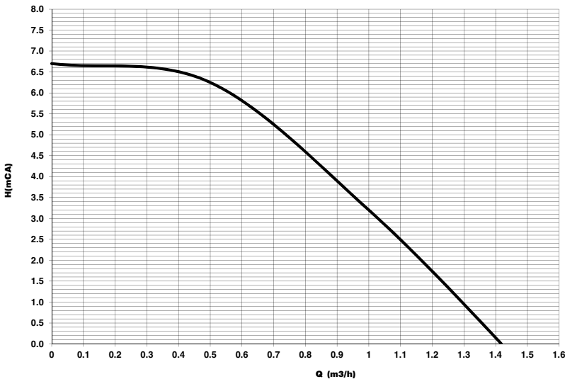
fig. 38 - Prevalenza residua disponibile all'impianto
