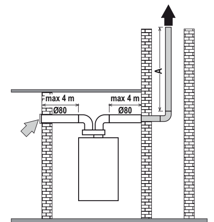
εικ. 24- Διάγραμμα μόνο για τοποθέτηση εύκαμπτου σωλήνα
