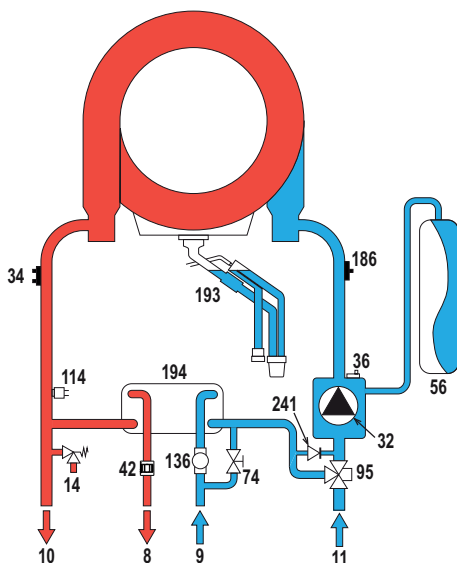
fig. 37 - Circuito idraulico
