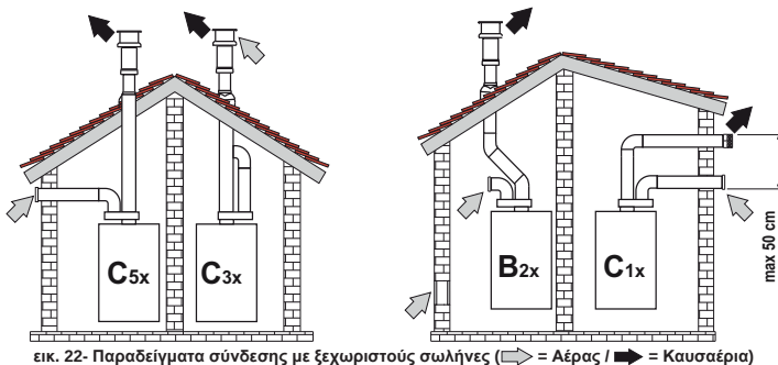
εικ. 22- Παραδείγματα σύνδεσης με ξεχωριστούς σωλήνες (⇐ = Αέρας / ➡ = Καυσαέρια)
