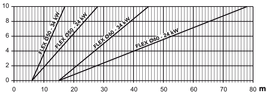
fig. 25 - Grafico per scelta parametro camino
