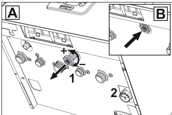
fig. 16- Filling knob
