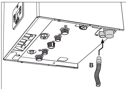
fig. 28- Racordarea evacuării condensului
