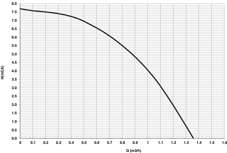
рис. 39- Остаточный напор, достигаемый в системе
