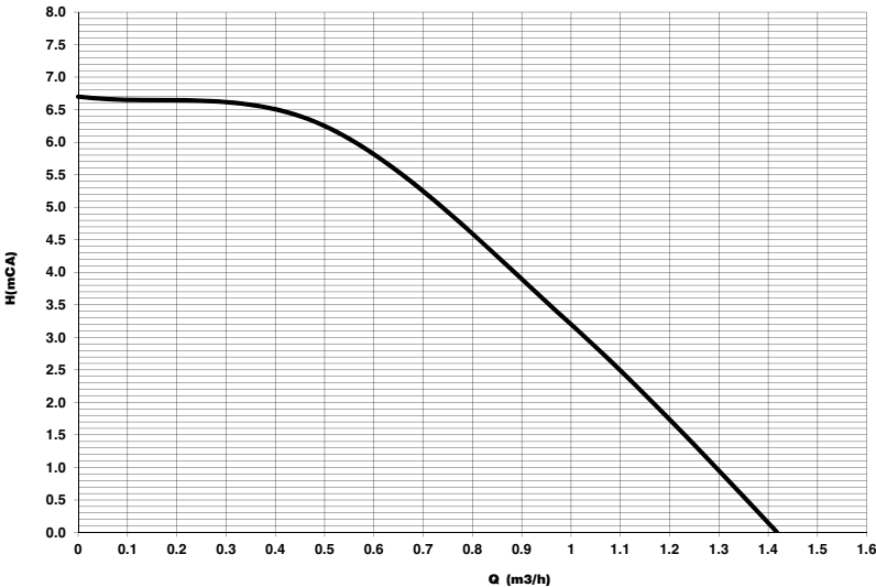
fig. 38- Carga hidrostática residual disponible en la instalación
