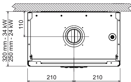
wygląd 34- Widok z góry
