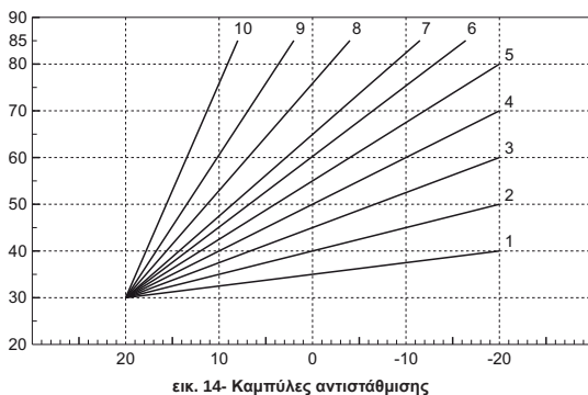
εικ. 14- Καμπύλες αντιστάθμισης
