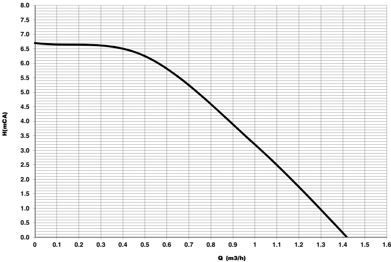
рис. 38- Остаточный напор, достигаемый в системе
