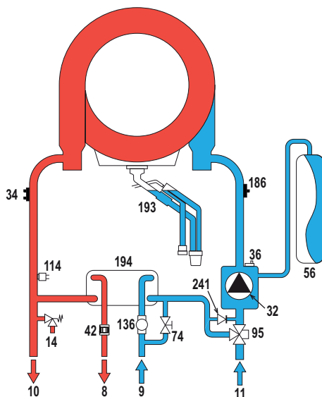
рис. 37- Гидравлический контур
