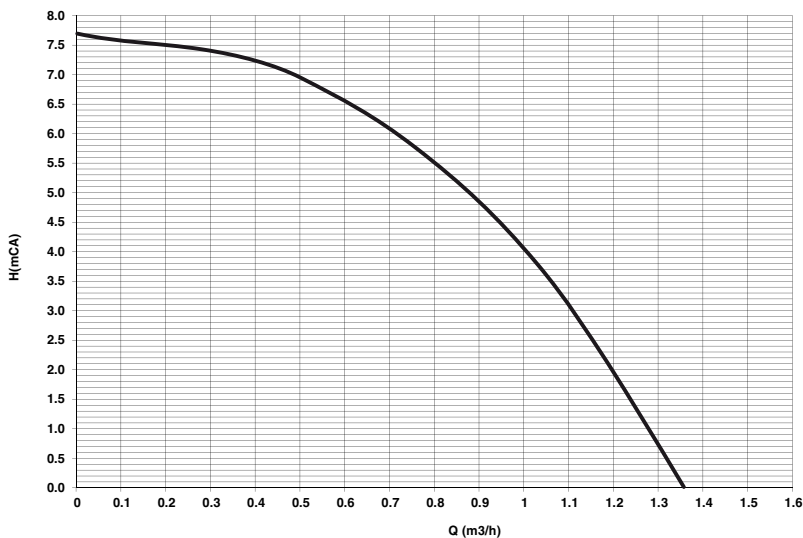
fig. 39- Înălțime de pompare reziduală disponibilă în instalație
