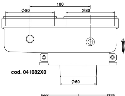
рис. 23- Исходная принадлежность для раздельных труб
