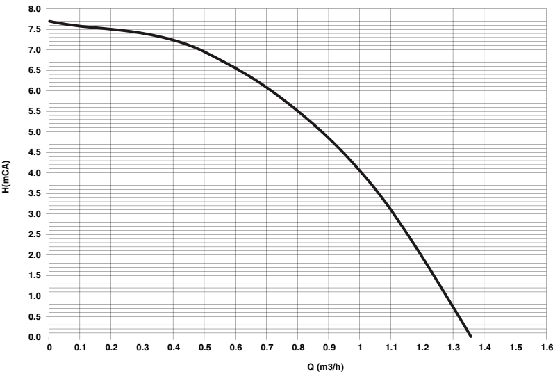
fig. 39- Carga hidrostática residual disponible en la instalación
