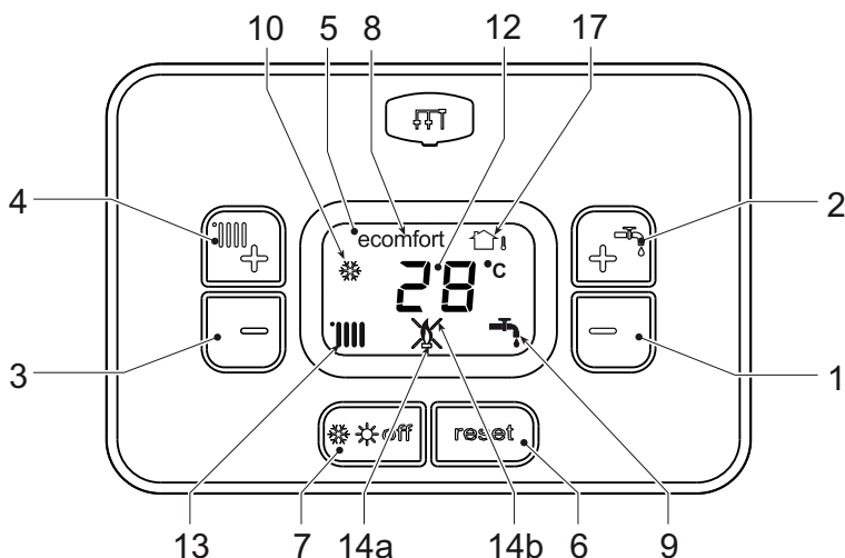
рис. 1- Панель управления
