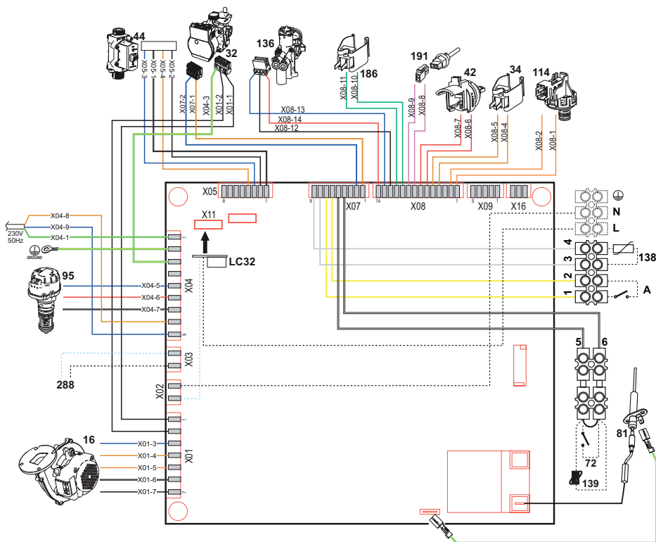
wygląd 40- Schemat elektryczny
