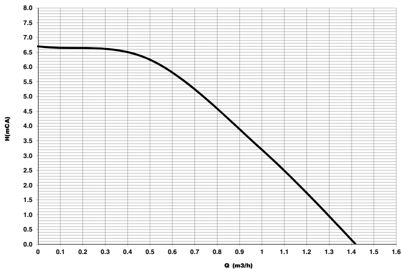
wygląd 38- Wysokość podnoszenia dostępna w instalacji
