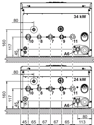
wygląd 35- Widok z dołu
