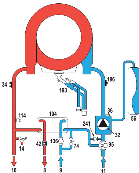
εικ. 37- Υδραυλικό κύκλωμα
