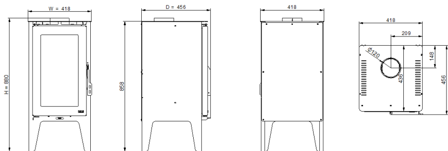
Figura 7 - Dimensiones de la estufa de leña Alva
