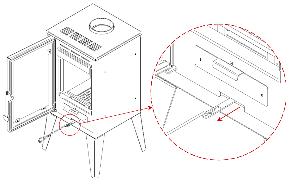
Figura 19 - Regulador de aire en posición abierta de aire primario
