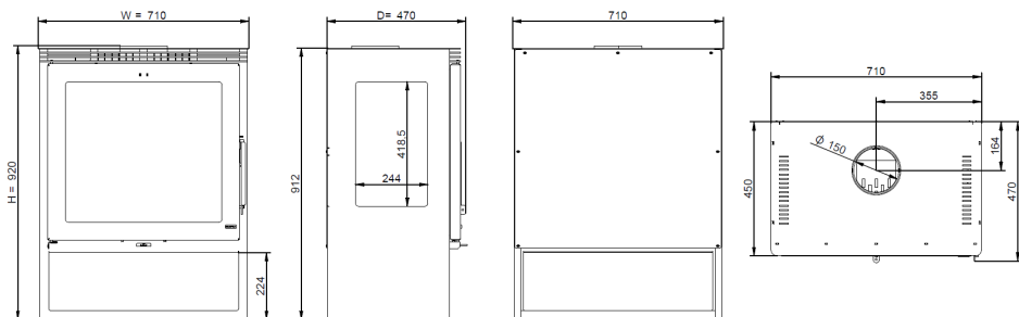
Figura 13 - Dimensiones de la estufa de leña Loire
