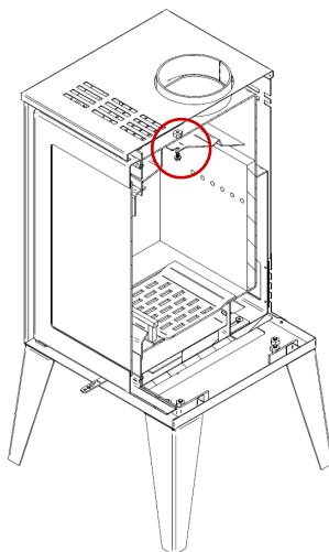
Figura 23 – Retire el segundo deflector
