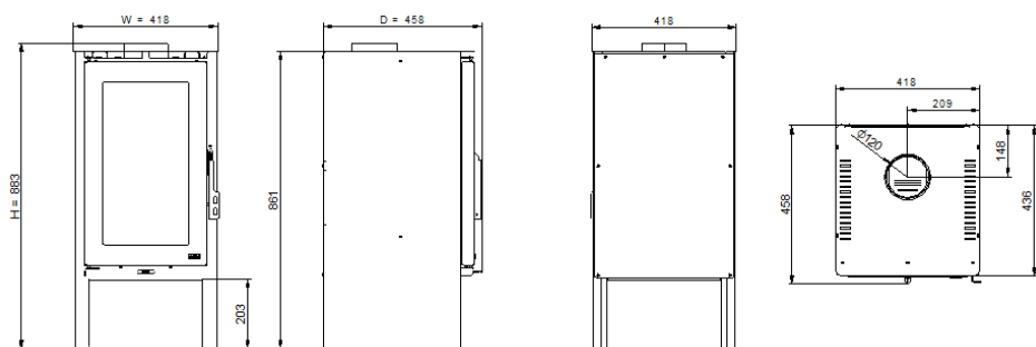
Figura 8 - Dimensiones de la estufa de leña Tejo
