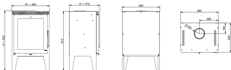
Figura 9 - Dimensiones de la estufa de leña Danúbio
