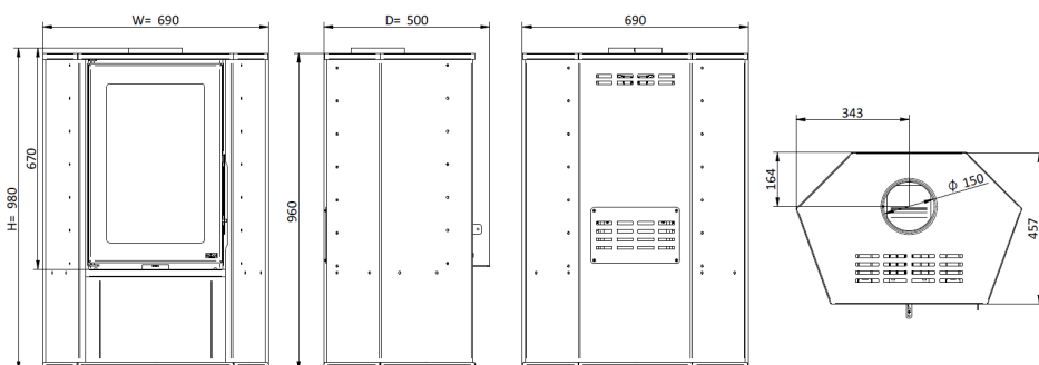
Figura 6 - Dimensiones de la estufa de leña Vizela
