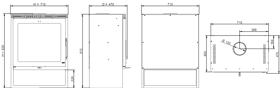
Figura 12 - Dimensiones de la estufa de leña Tibre
