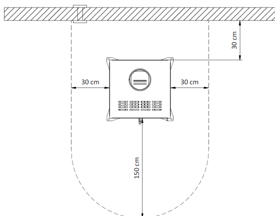
Figura 18 - Distancias mínimas de seguridad
