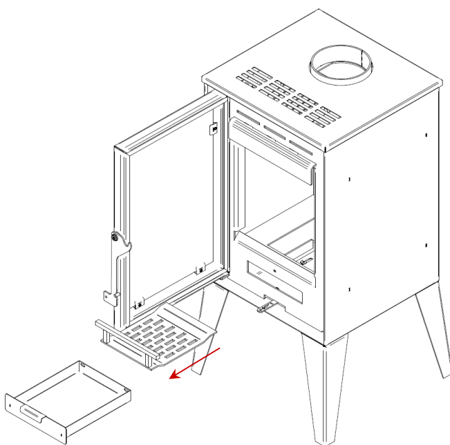
Figura 21 – Limpieza del cajón de las cenizas
