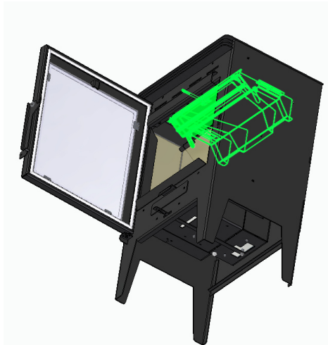
Figura 25 – Retire el segundo deflector
