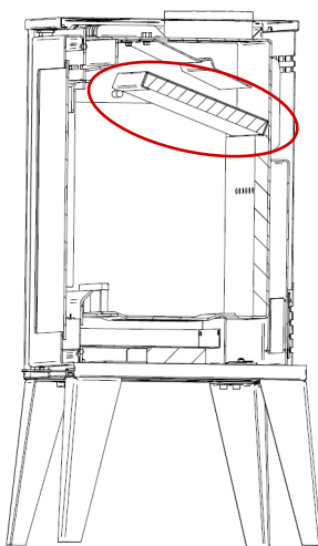
Figura 22 – Retire el primer deflector
