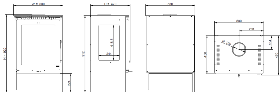
Figura 14 - Dimensiones de la estufa de leña Sena
