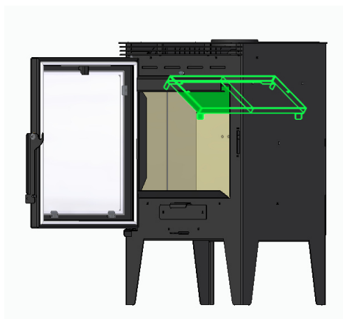
Figura 24 – Retire el primer deflector
