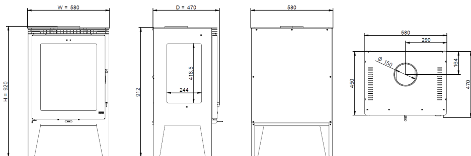
Figura 11 - Dimensiones de la estufa de leña Reno
