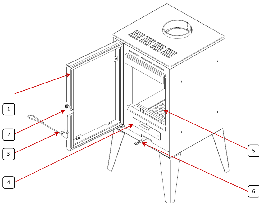
Figura 15 - Componentes de la estufa
