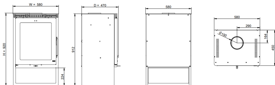
Figura 10 - Dimensiones de la estufa de leña Nilo
